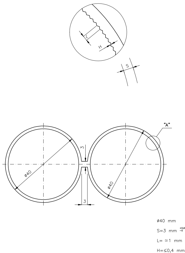
FIGURA N° 1: SECCION DE BITUBO PEHD \phi 40 mm
