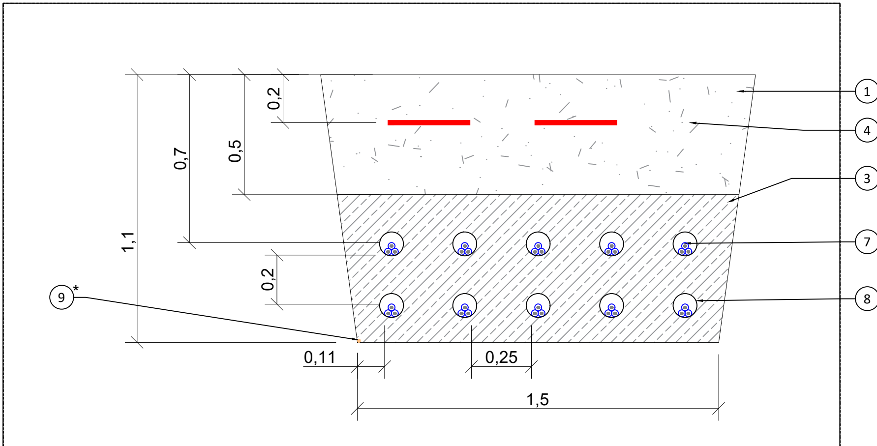
TIPO IV MAX 10 CIRCUITOS CABLE BT (Al) EN TUBO BAJO CAMINO
