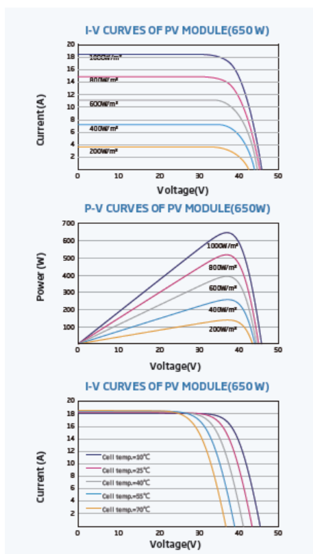
Ilustración 12. Curvas características
