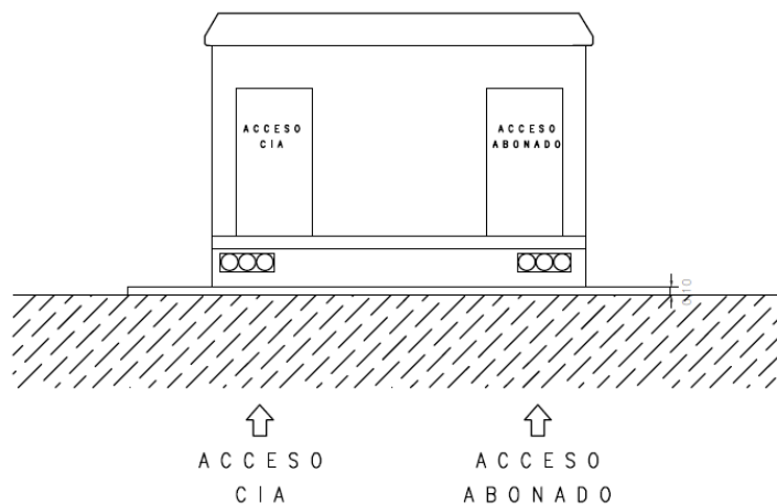
Ilustración 21. Alzado CPM
