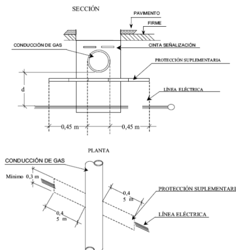
Ilustración 28. Detalles de cruzamiento y conducciones (ITC-LAT 06)
