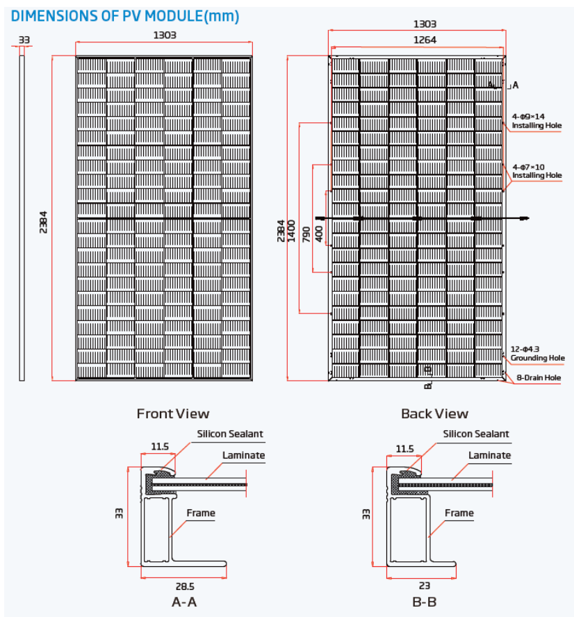
Ilustración 11. Módulo fotovoltaico
