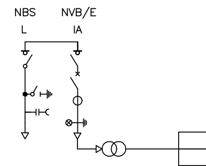
ESQUEMA UNIFILAR
