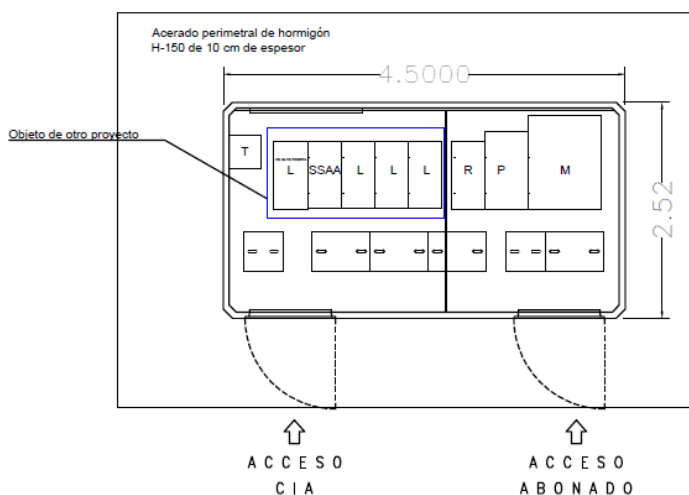
Ilustración 22. Planta CPM
