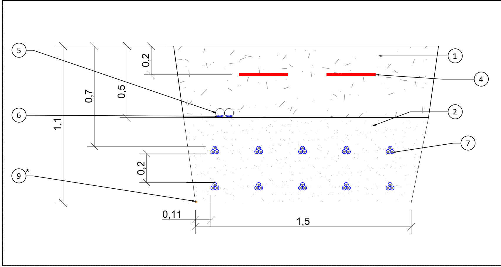
TIPO II MAX 2 TUBOS PARA CABLE SOLAR (Cu) MAX 10 CIRCUITOS CABLE BT (Al)
