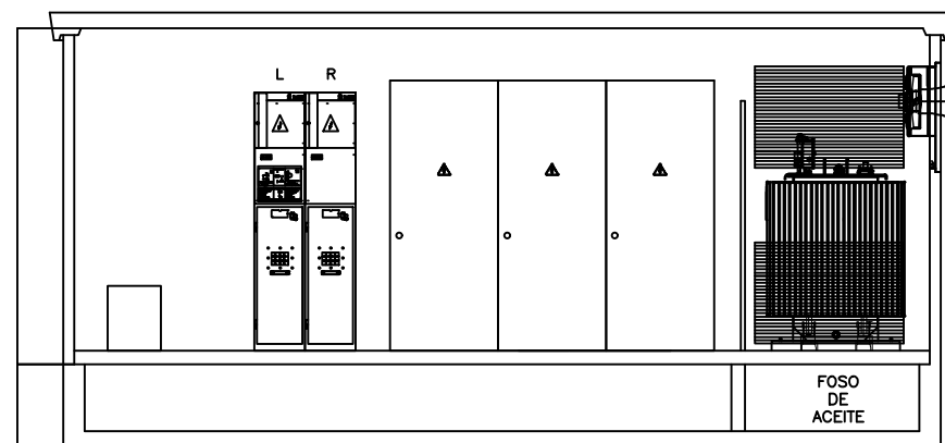
SECCION LONGITUDINAL
