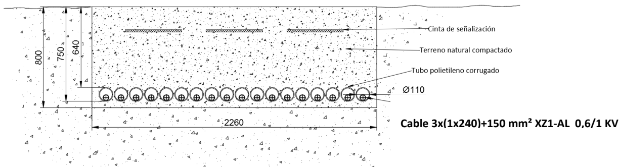
Ilustración 8.3 - Doc. I. Memoria - Detalle zanja BT. Paso a bajo tubo.
