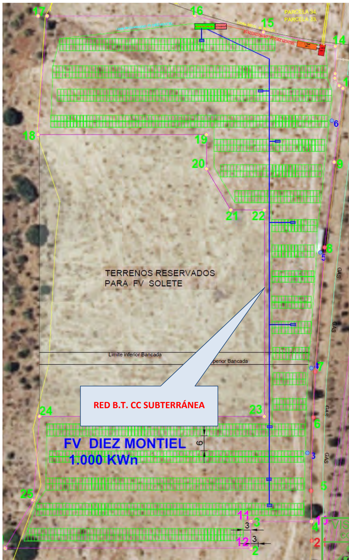
Ilustración 9.3 - Doc. I. Trazado Línea Subterránea BT de evacuación
