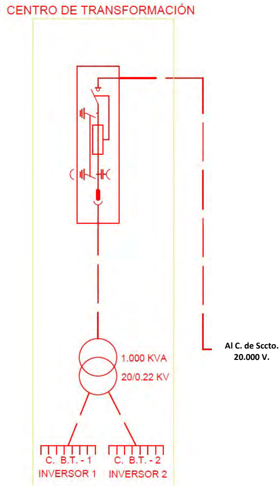
Ilustración 9.2 - Doc. I. Memoria - Esquema eléctrico del Centro de Transformación
