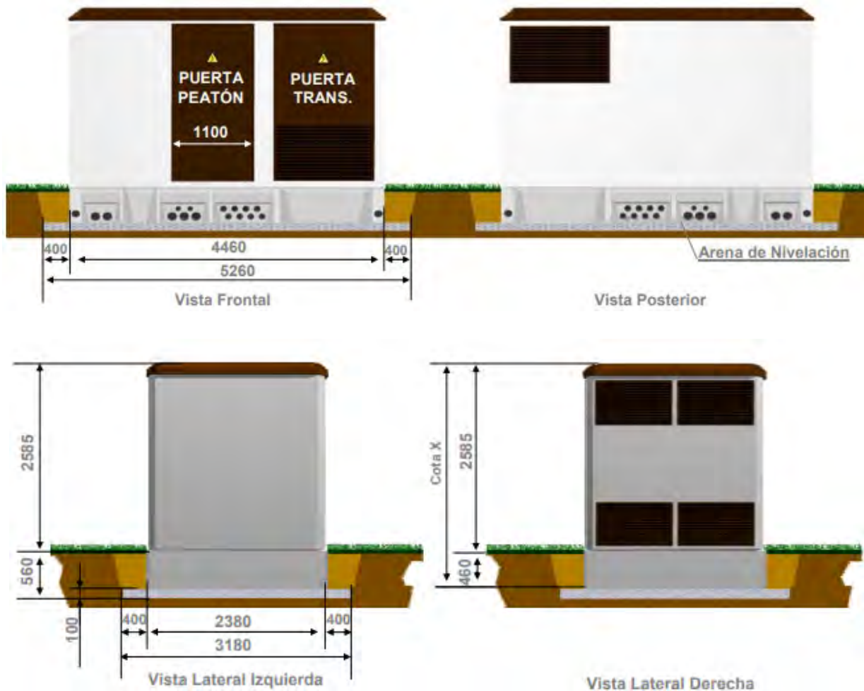
Ilustración 8.6 - Doc. I. Memoria – Edificio prefabricado pfu-4/20 para el Centro de transformación
