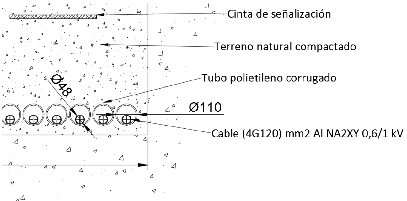
Ilustración 5.1 - Doc. II. Cálculos - Dimensiones canalizaciones BT.
