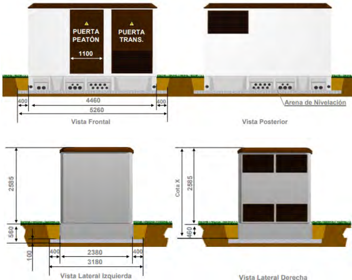
Ilustración 8.6 - Doc. I. Memoria – Edificio prefabricado pfu-4/20 para el Centro de transformación
