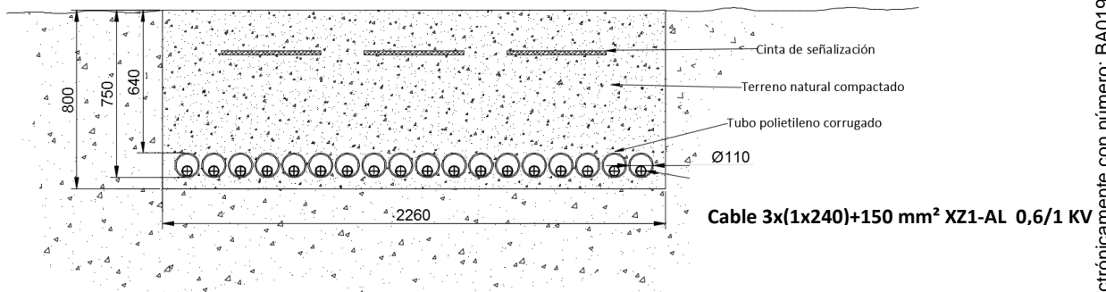
Ilustración 8.3 - Doc. I. Memoria - Detalle zanja BT. Paso a bajo tubo.
