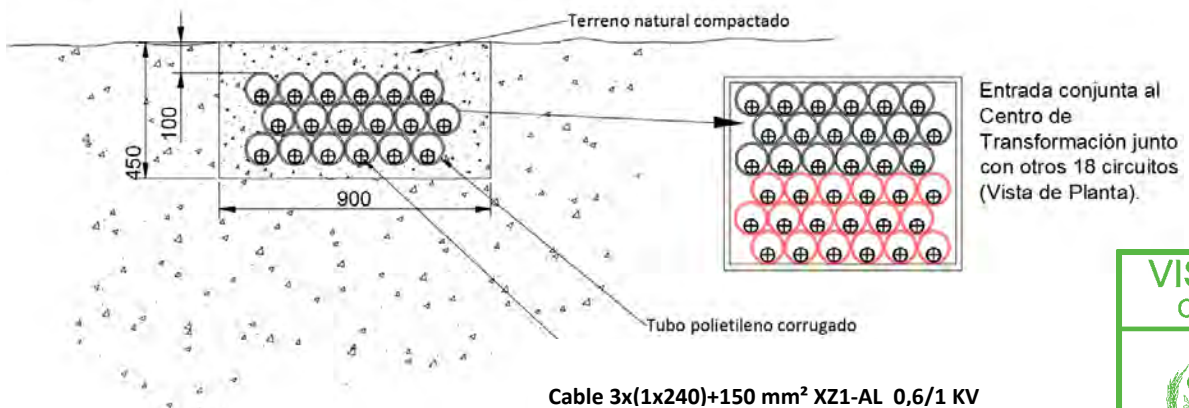
Ilustración 8.4 - Doc. I. Memoria - Detalle zanja BT. Acometiendo a CT.
