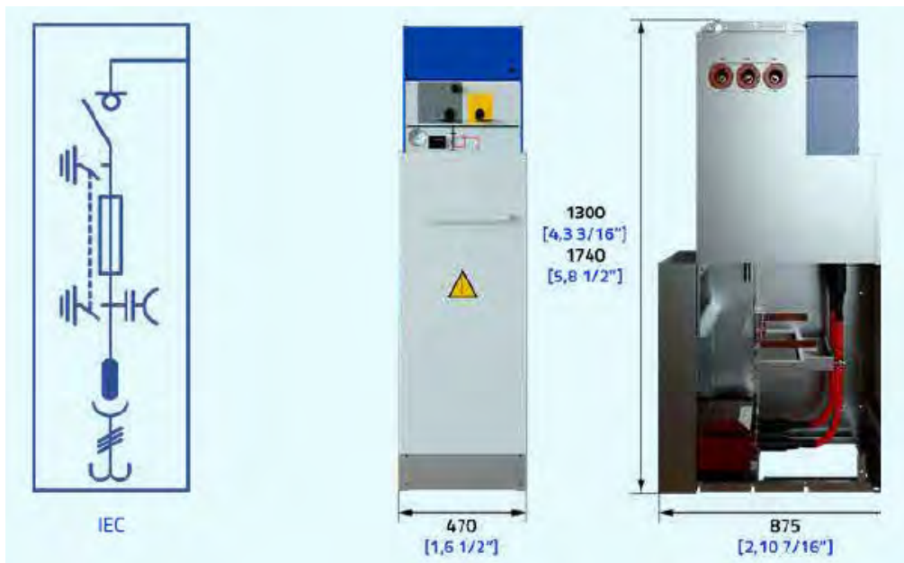
Ilustración 11.4 - Doc. I. Memoria – Celda de Servicios Auxiliares con transformador de 600 VA. 20/B2
