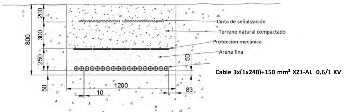
Ilustración 8.2 - Doc. I. Memoria - Detalle zanja BT. Cables directamente enterrados.
