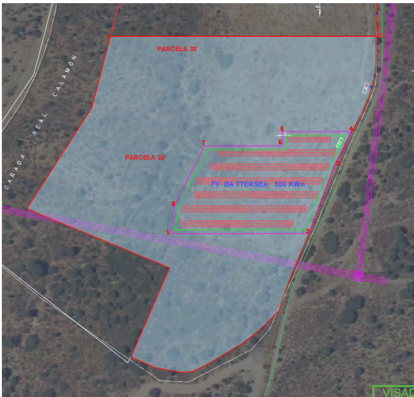
Ilustración 7. - Doc. I. Memoria – Poligonal de la Instalación e Implantación de Módulos (Magenta) y Parcela (Rojo)
