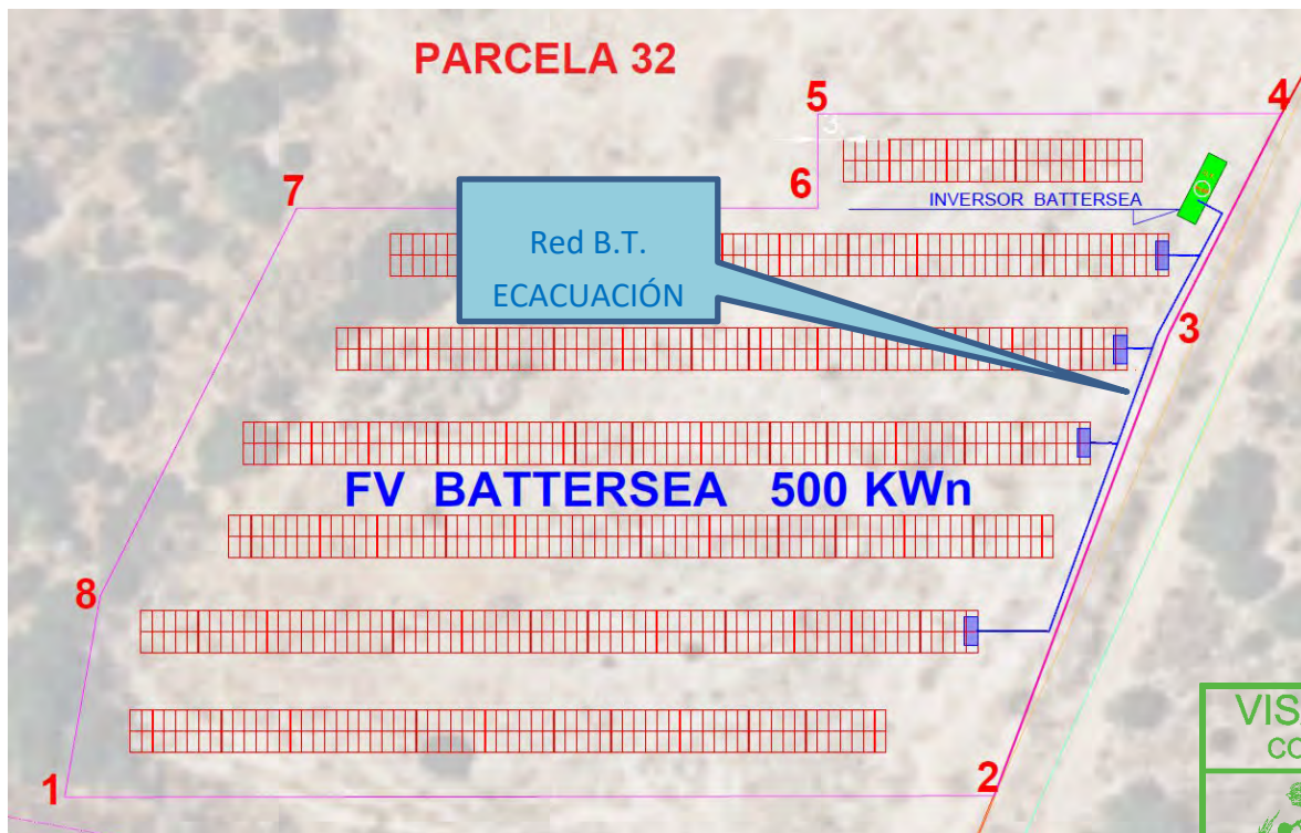
Ilustración 9.3 - Doc. I. Trazado Línea Subterránea BT de evacuación
