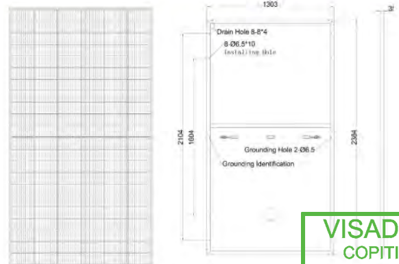
Ilustración 8.1 - Doc. I. Memoria. Características físicas MODULO FOTOVOLTAICO. TAMESOL TM-650/670M-132HC
