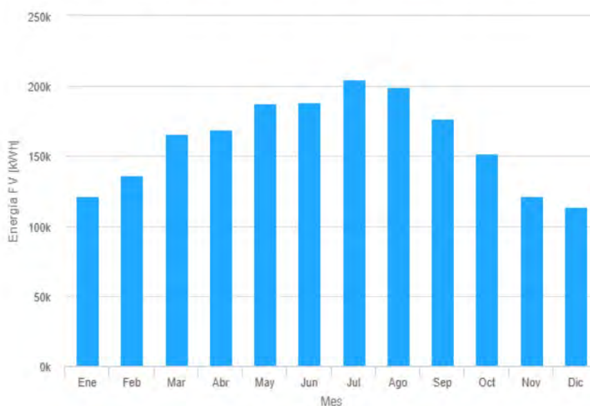
Producción de energía mensual del sistema FV fijo:
