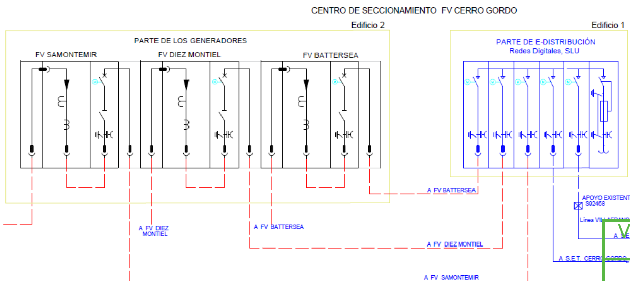
Ilustración 11.3 - Doc. I. Memoria – Esquema unifilar del Centro de Seccionamiento, completo
