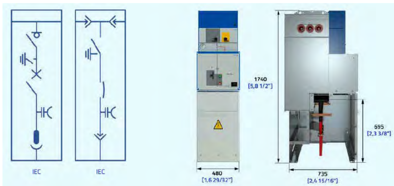
Ilustración 11.5 - Doc. I. Memoria – Celda prefabricada de INTERRUOTIR AUTOMÁTICO DE VACÍO.
