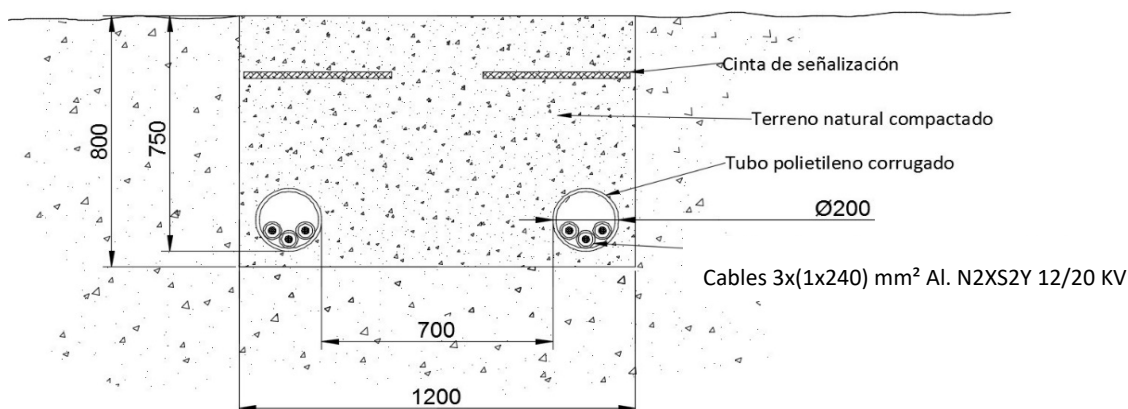
Zanja Tipo 6. Conexión entre Centros de Transformación (Acometiendo a CT)
