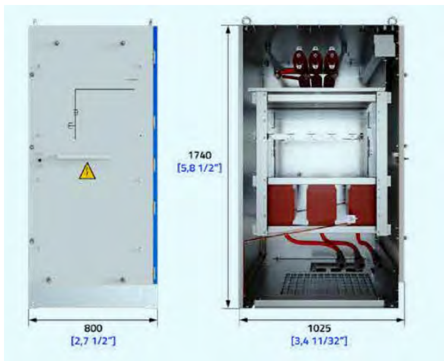
Ilustración 11.20 - Doc. I. Memoria – Celda prefabricada de MEDIDA.
