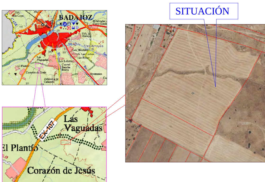
Ilustración 6.1. - Doc. I. Memoria - Situación de la planta FV.
