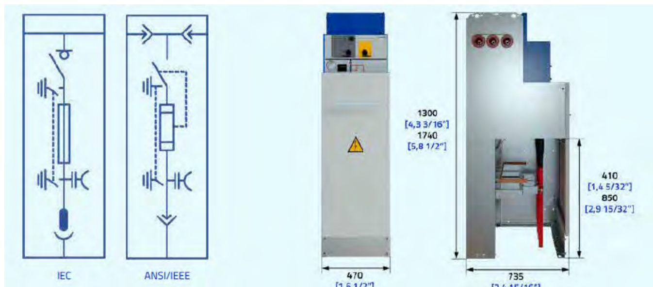
Ilustración 9.15 - Doc. I. Memoria – Celda prefabricada de Protección de Transformador
