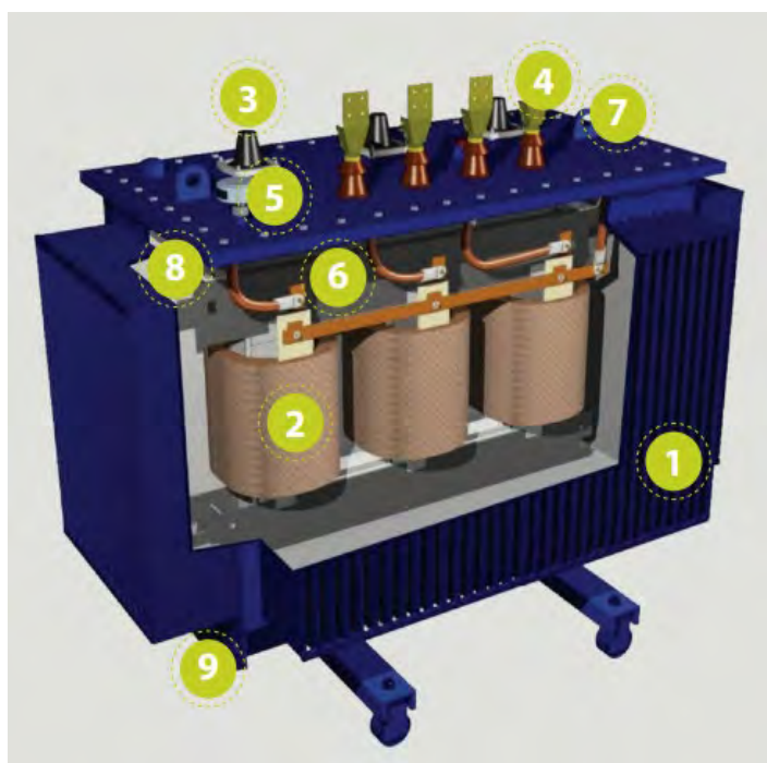
Ilustración 9.16 - Doc. I. Memoria – Sección y elementos fundamentales del Transformador
