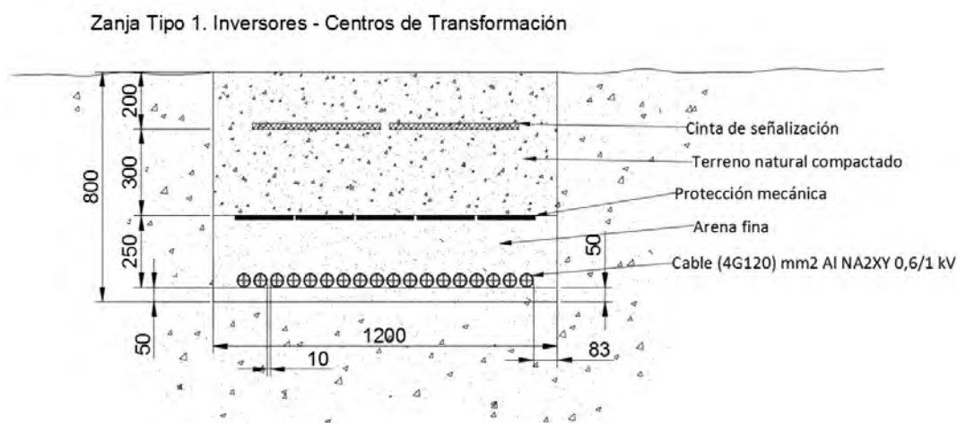
Ilustración 16.2 - Doc. I. Memoria - Detalle zanja BT. Cables directamente enterrados.
