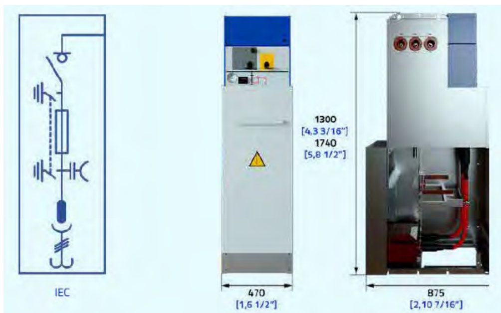
Ilustración 11.18 - Doc. I. Memoria – Celda de Servicios Auxiliares con transformador de 600 VA. 20/B2
