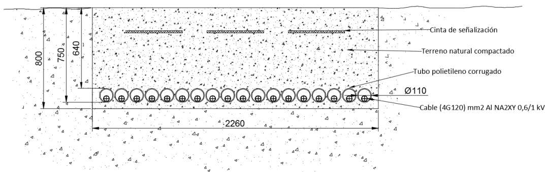
Ilustración 16.3 - Doc. I. Memoria - Detalle zanja BT. Paso a bajo tubo.
