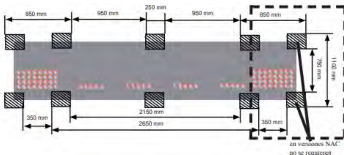
Ilustración 8.4 - Doc. I. Memoria. Cimentación de apoyo del INVERSOR
