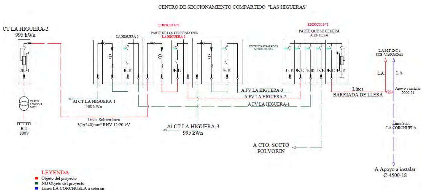
Ilustración 11.17 - Doc. I. Memoria – Esquema unifilar del Centro de Seccionamiento, completo
