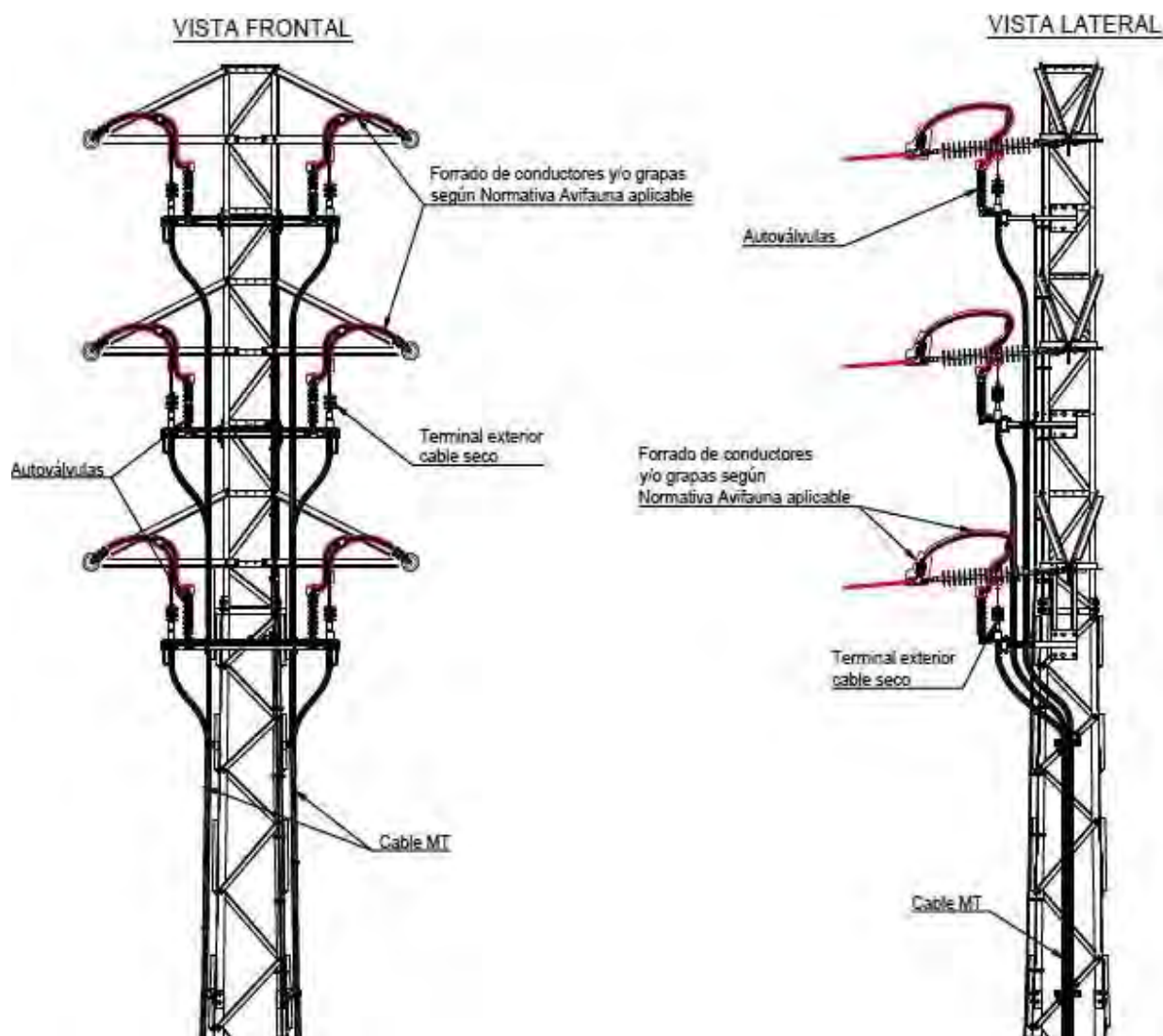
Ilustración 15.22 - Doc. I. Memoria. Detalles de la cabeza del apoyo A-410635 con el Paso a Subterránea de la línea D/C
