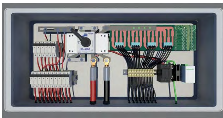
Ilustración 8.6 - Doc. I. Memoria. Caja de Agrupamiento.
