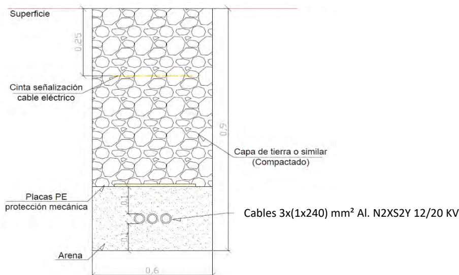
Ilustración 12.1 - Doc. I. Memoria - Detalle Zanja MT. Cables directamente enterrados. SIMPLE CIRCUITIO
