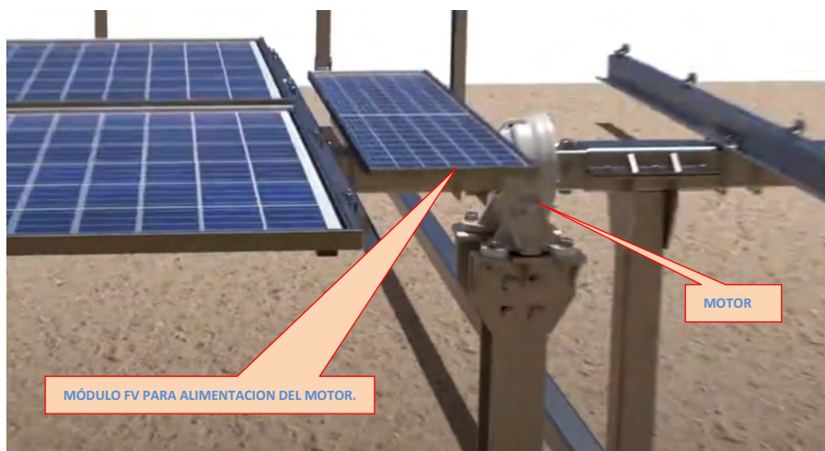
Ilustración 8.9 - Doc. I. Memoria. Módulo FV para la alimentación del Motor del seguidor.
