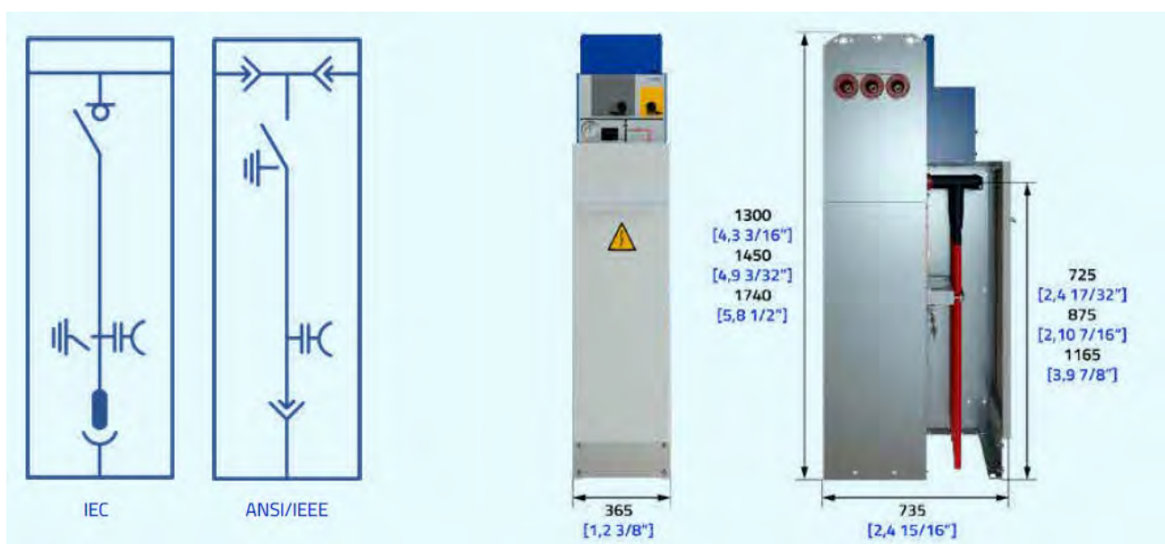
Ilustración 11.3 - Doc. I. Memoria – Celda de Servicios Auxiliares con transformador de 600 VA. 20/B2
