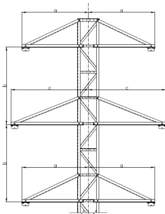
Ilustración 15.3 - Doc. I. Memoria. Detalles de la cabeza del apoyo A-410635 con el Paso a Subterránea de la línea.
