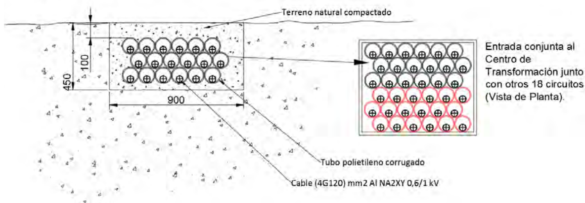
Ilustración 16.4 - Doc. I. Memoria - Detalle zanja BT. Acometiendo a CT.
