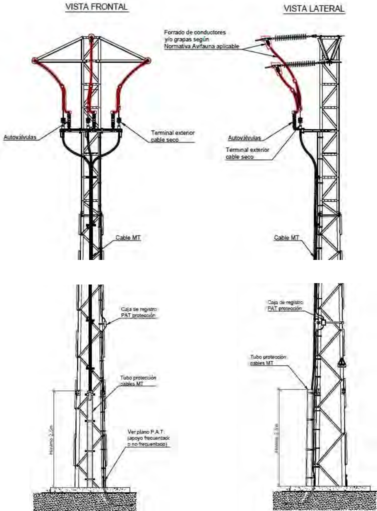
Ilustración 15.24 - Doc. I. Memoria. Detalles de la cabeza y base del apoyo A-410635 con el Paso a Subterránea de la línea.
