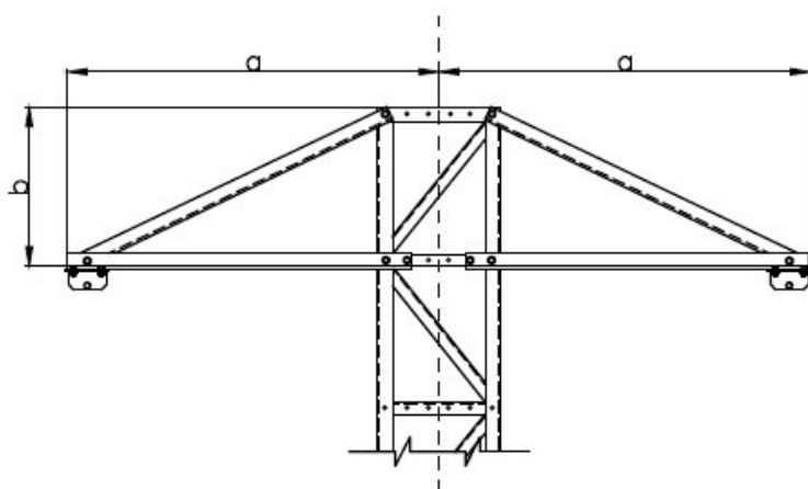
Ilustración 15.23 - Doc. I. Memoria. Detalles de la cabeza del apoyo A-410635 con el Paso a Subterránea de la línea.
