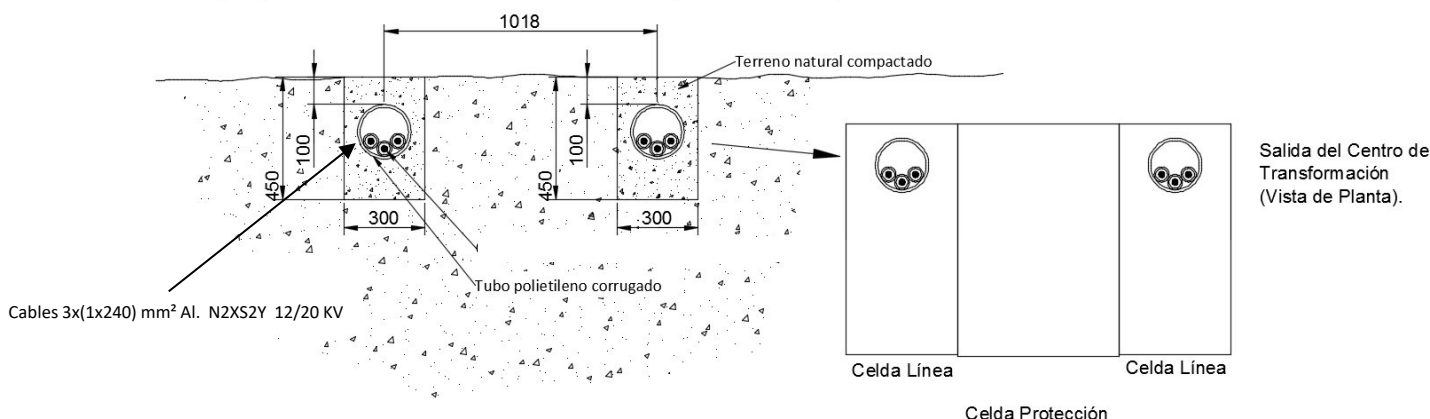
Ilustración 16.7 - Doc. I. Memoria. Tipos de Zanja para Línea Subterránea MT D/C, 20kV
