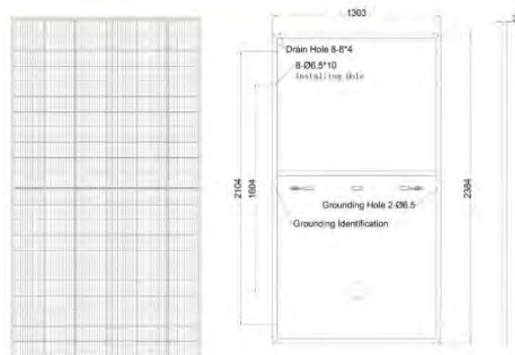
Ilustración 8.1 - Doc. I. Memoria. Características físicas MODULO FOTOVOLTAICO. TAMESOL TM-650/670M-132HC
