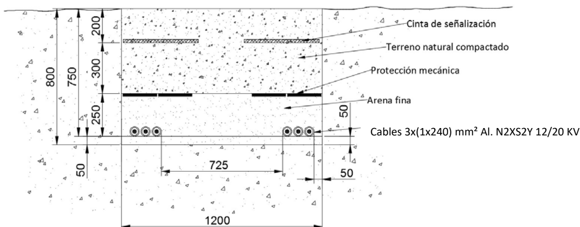
Ilustración 16.5 - Doc. I. Memoria. Tipo de Zanja, para línea Subterránea MT D/C, 20kV
