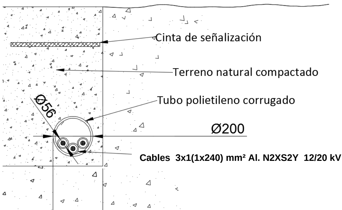
Ilustración 5.2 - Doc. II. Cálculos - Dimensiones canalizaciones AT.
