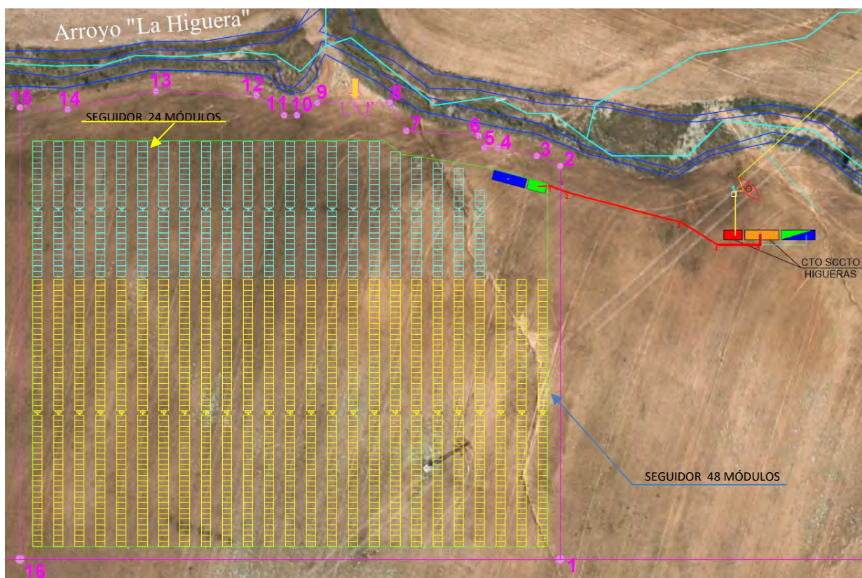
Ilustración 6.3 - Doc. I. Memoria. IMPLANTACIÓN PREVISTA de la planta FV. LA HIGUERA-2
