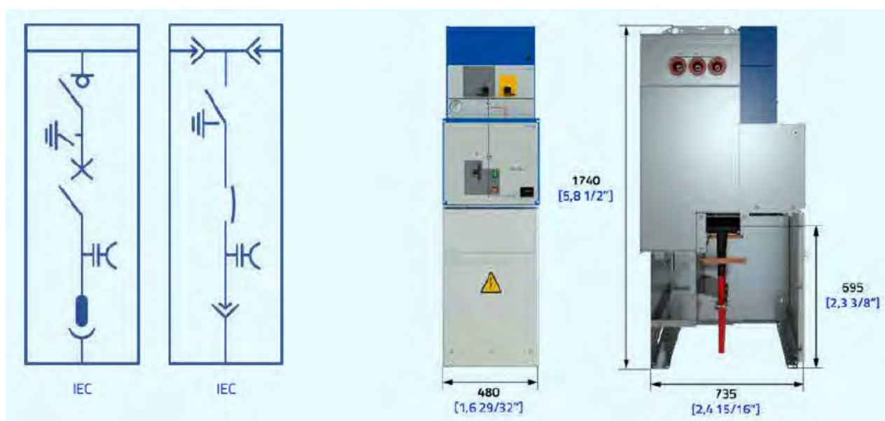
Ilustración 11.19 - Doc. I. Memoria – Celda prefabricada de INTERRUOTIR AUTOMÁTICO DE VACÍO.
