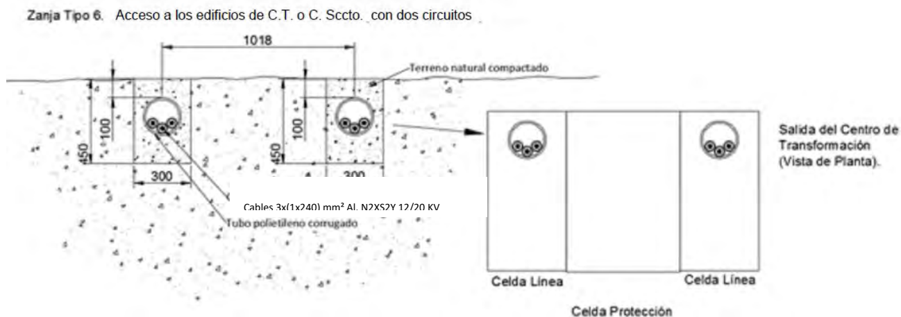
Ilustración 16.7 - Doc. I. Memoria. Tipos de Zanja para Línea Subterránea MT D/C, 20kV
