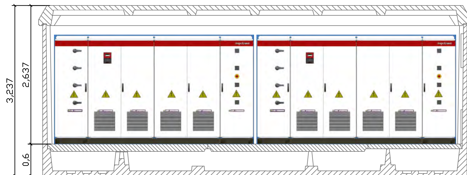
VISTA POSTERIOR
