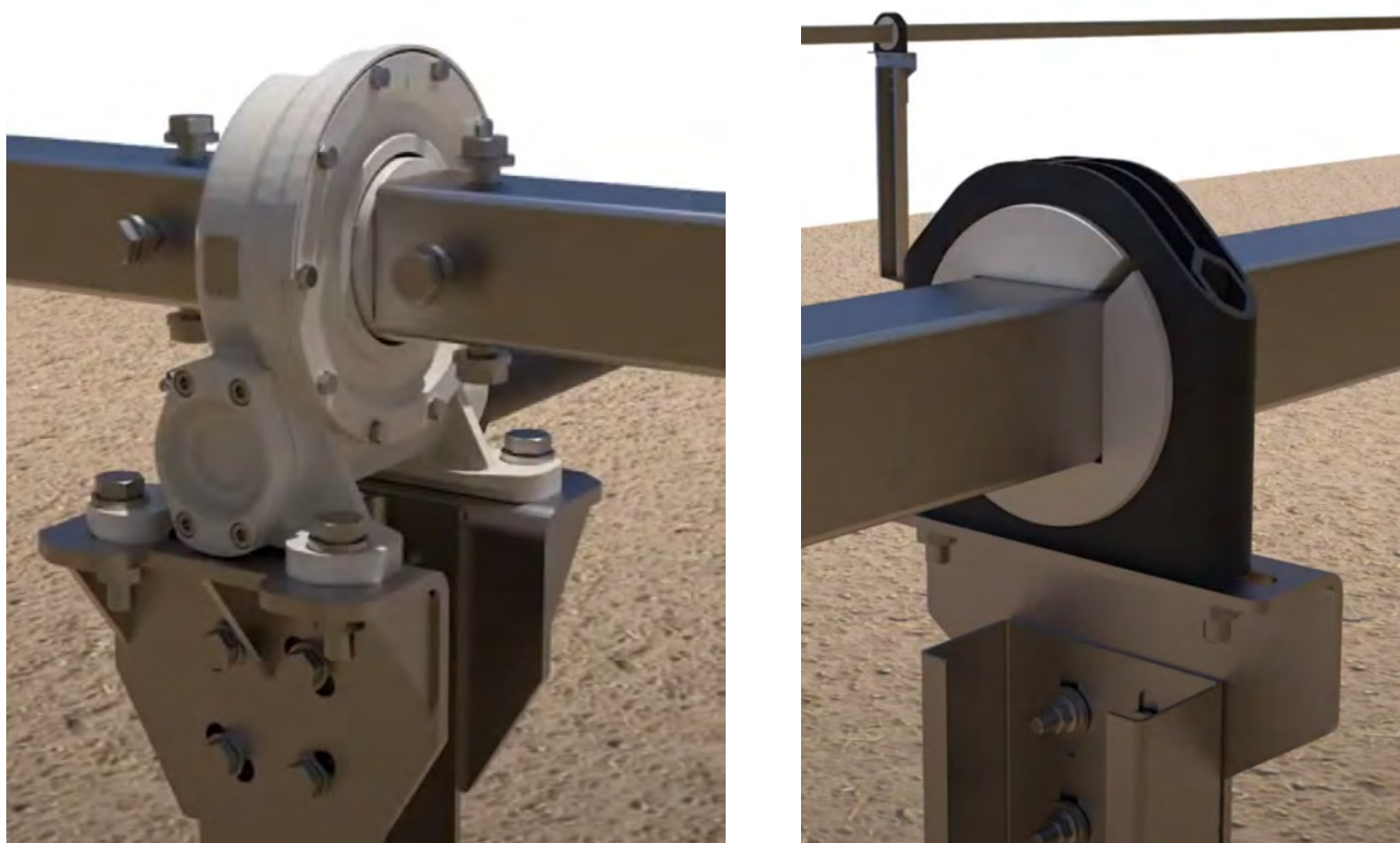
Ilustración 8.5 - Doc. I. Memoria. Motor y Rótula instalada en el seguidor
