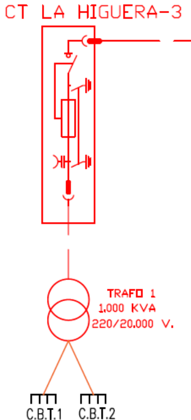
Ilustración 7.10 - Doc. I. Memoria - Esquema eléctrico del Centro de Transformación FV LA HIGUERA-3
