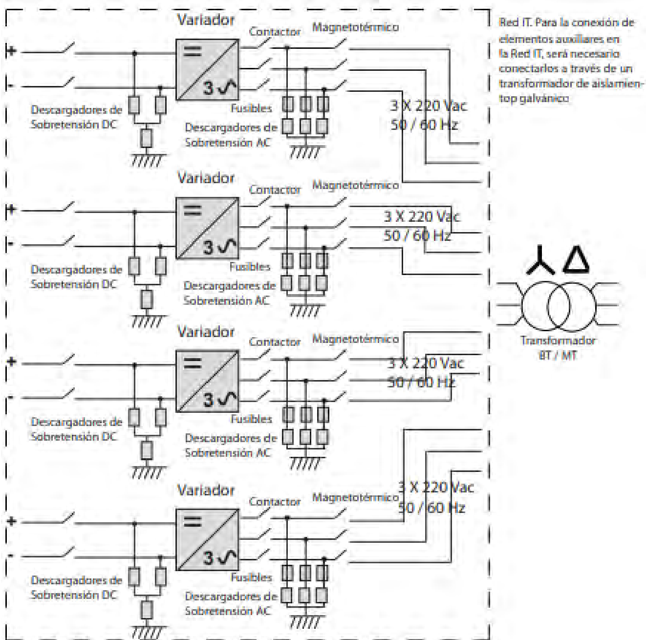
Ilustración 8.3 - Doc. I. Memoria. Esquema unifilar del INVERSOR
