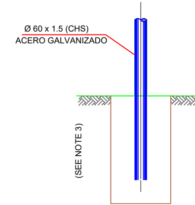
DETALLE ENCOFRADO
