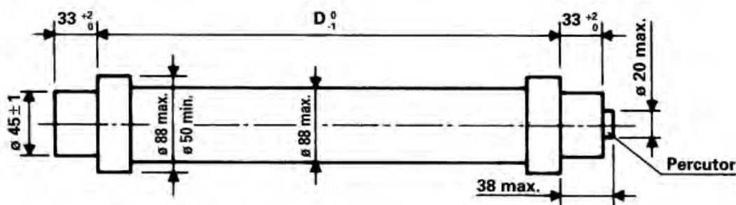
Fig. 1: fusible limitador
