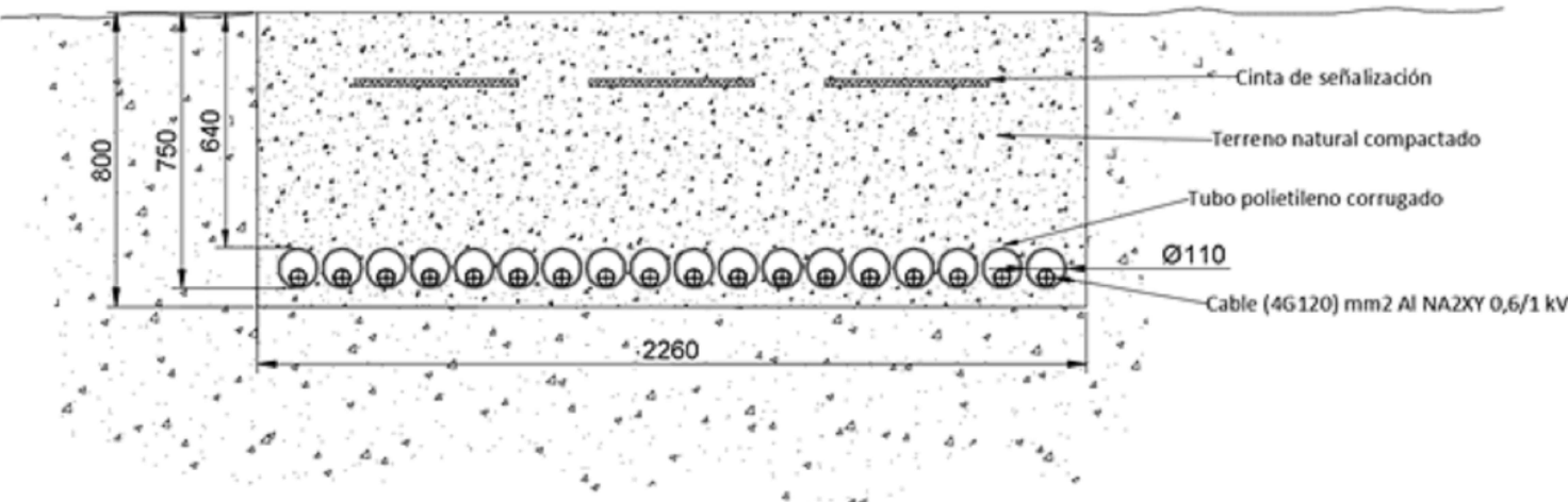
Zanja Tipo 2. Inversores - Centros de Transformación (Paso a bajo tubo)
