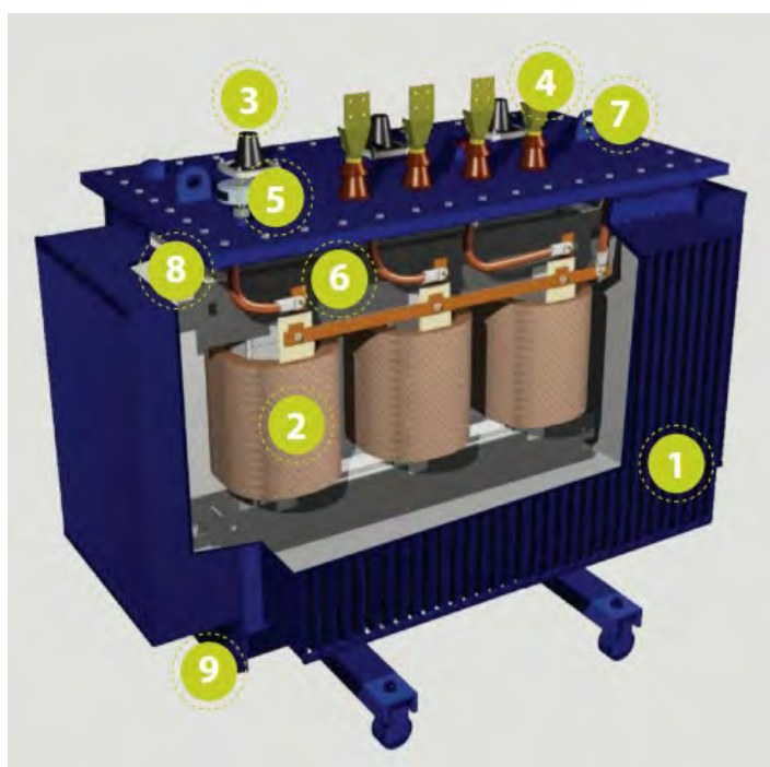
Ilustración 9.11 - Doc. I. Memoria – Sección y elementos fundamentales del Transformador
