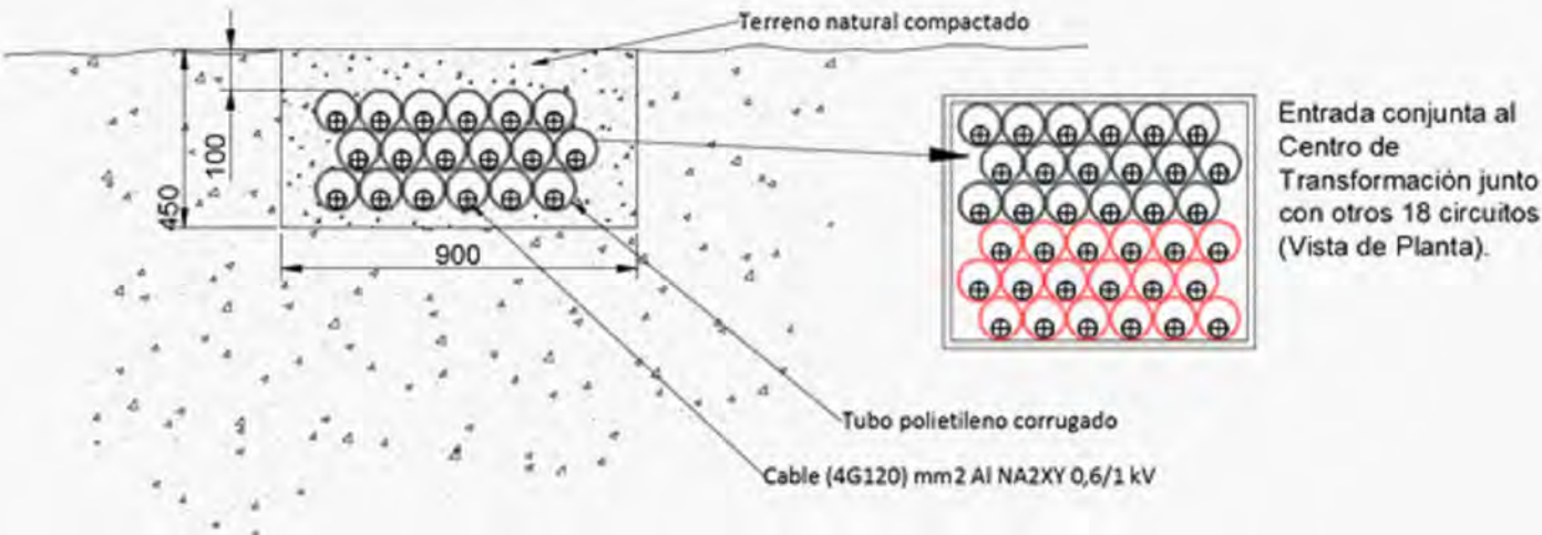
Zanja Tipo 3. Inversores - Centros de Transformación (acometiendo al CT)
