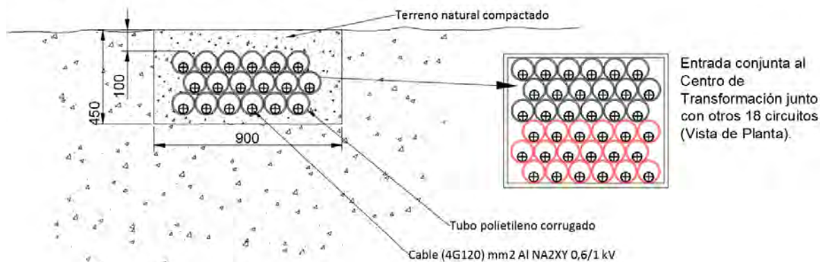
Ilustración 13.5.1.3 - Doc. I. Memoria - Detalle zanja BT. Acometiendo a CT.
