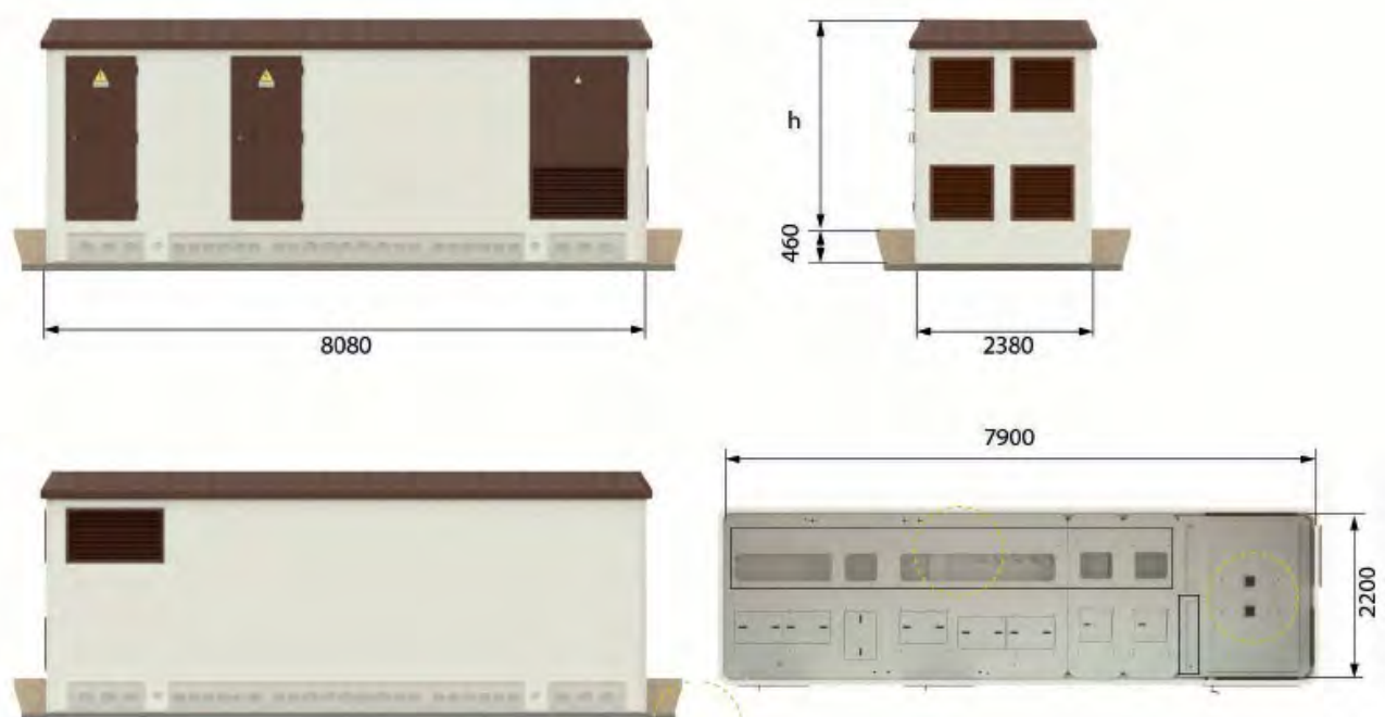
Ilustración 10.13.1 - Doc. I. Memoria – Edificio prefabricado pfu-7/20 para el Centro de inversores Y Edificio 2 de SCCTO
