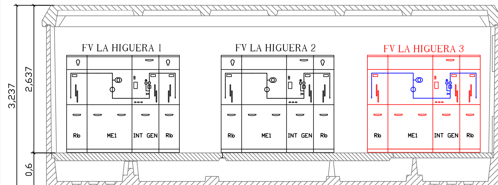
VISTA POSTERIOR
