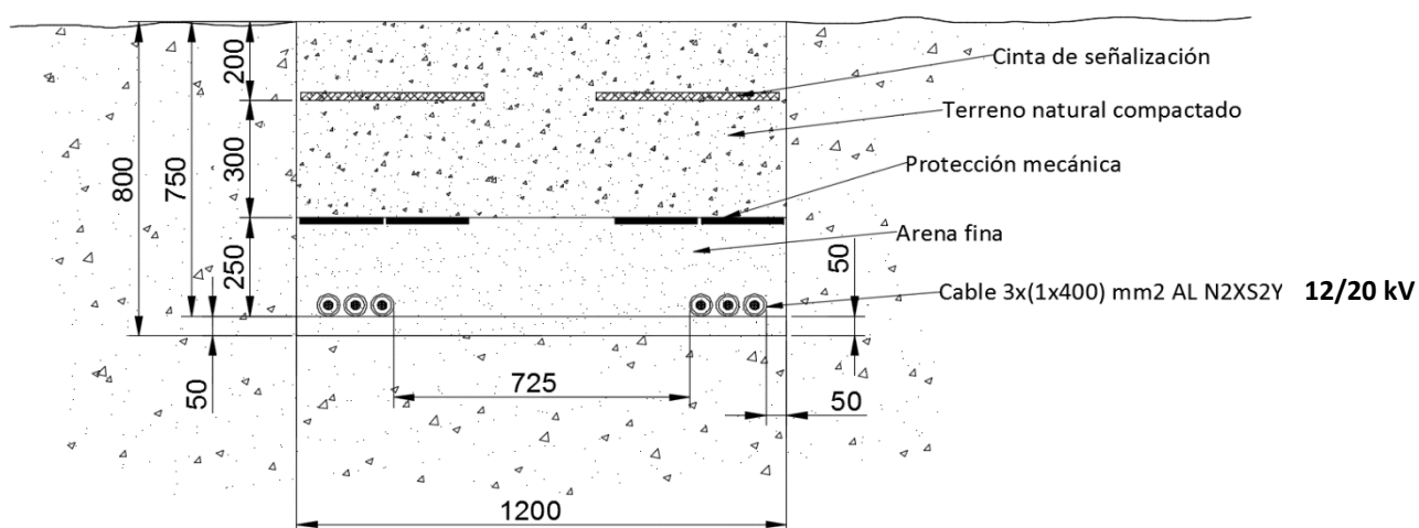
Zanja Tipo 4. Conexión entre Centros de Transformación
