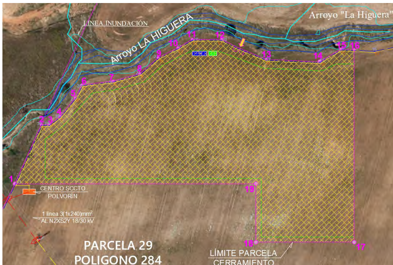
Ilustración 6.2.3 - Doc. I. Memoria - POLIGONAL de las Parcela donde se ubica PLANTA FV
