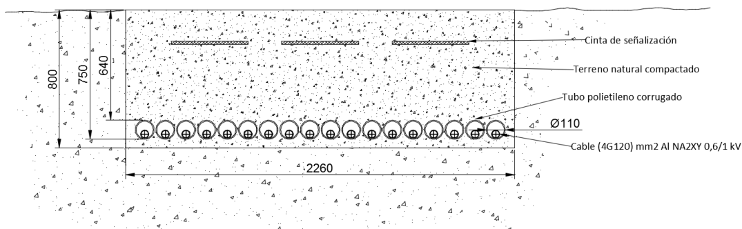
Ilustración 13.5.1.2 - Doc. I. Memoria - Detalle zanja BT. Paso a bajo tubo.
