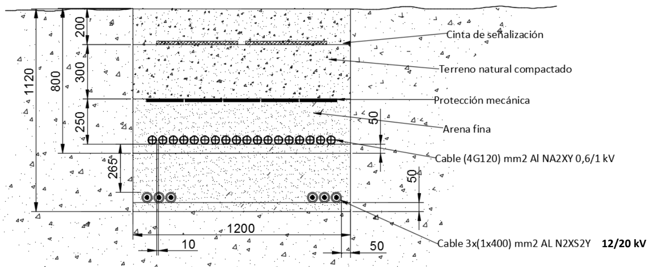
Zanja Tipo 8. Tramos coincidentes Zanja Tipo 1 y 4.
