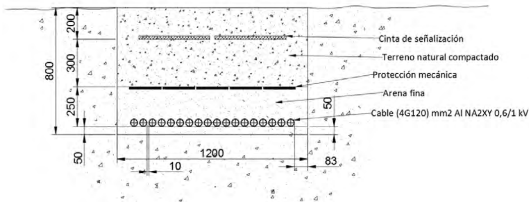
Ilustración 13.5.1.1 - Doc. I. Memoria - Detalle zanja BT. Cables directamente enterrados.
