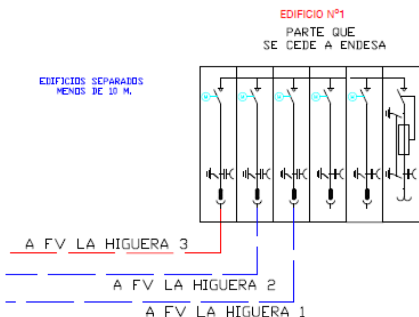
Ilustración 7.8.2 - Doc. I. Memoria – Esquema unifilar del Centro de Seccionamiento, parte de Endesa.
