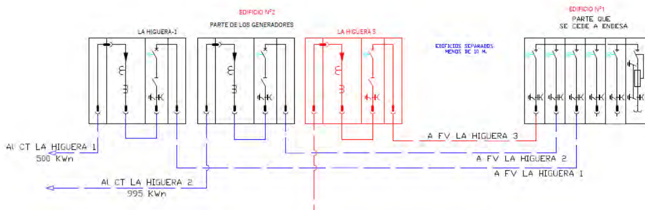
Ilustración 11.12 - Doc. I. Memoria – Esquema unifilar del Centro de Seccionamiento, completo
