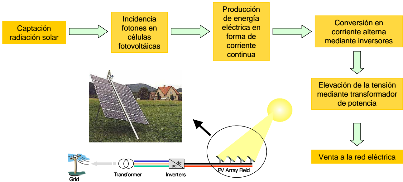
Figura 20: Principio de Funcionamiento Instalación FV.
