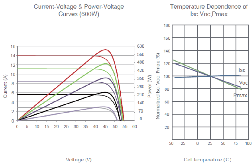
Figura 23: Curvas Características JKM600N-78HL4.
