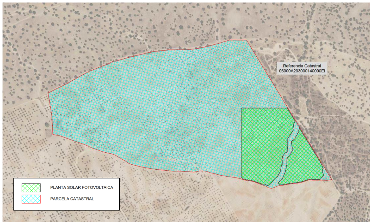
Figura 4: Área disponible para la Implantación de la Planta Solar FV.
