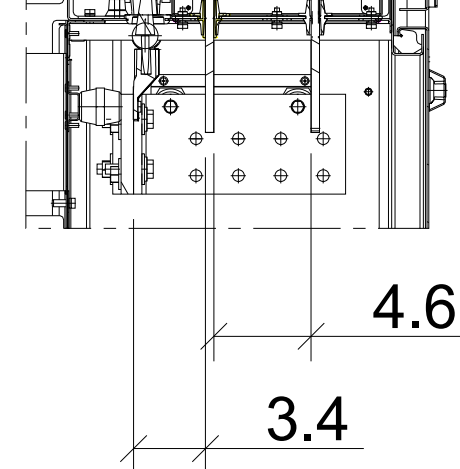
E (1:15)
