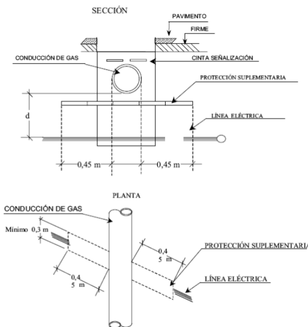
Figura 29: Detalles de cruzamiento y conducciones (ITC-LAT 06).
