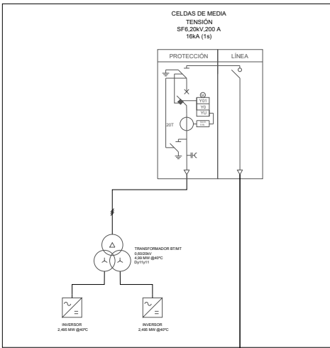
SKID MT TIERRA DE BADAJOZ 3
