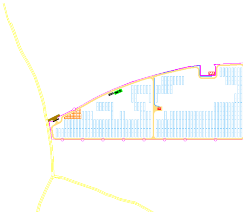
Figura 21: Planta Solar FV.
