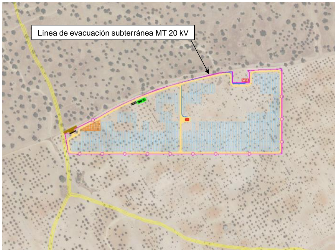
Figura 25: Localización LSMT 20 kV
