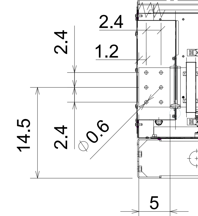
A (1:15)
