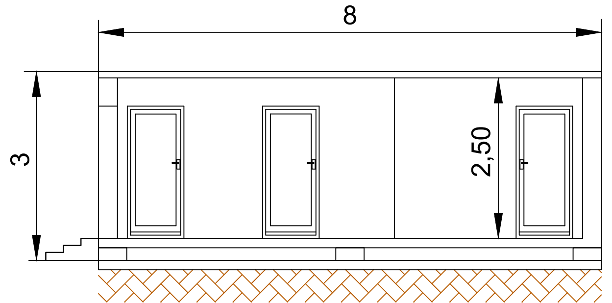
SECCIÓN A-A'
