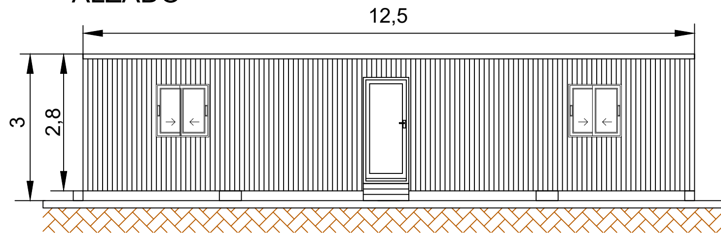
ALZADO
