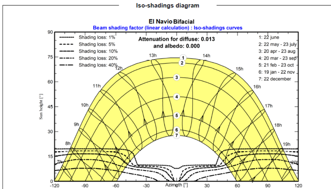
Ilustración 5. Diagrama de Iso-sombreados
