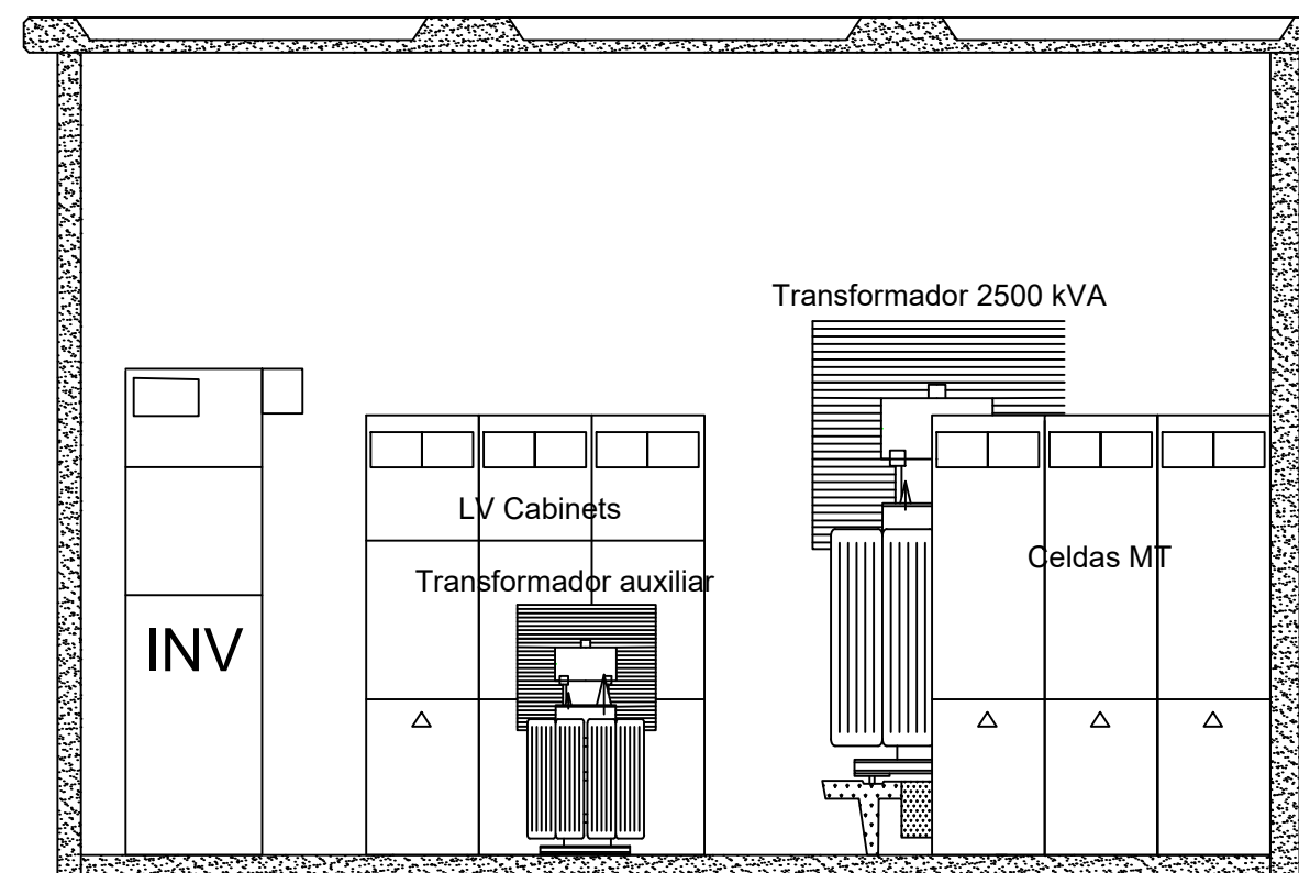
SECCIÓN A-A'
