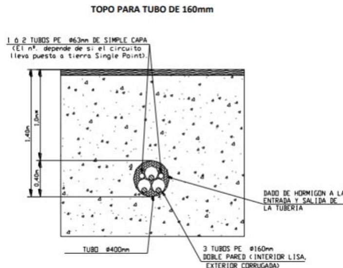
Ilustración 9. Topo
