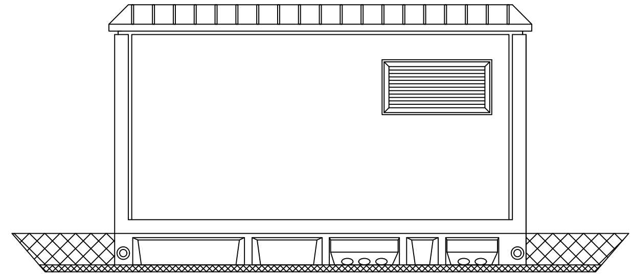
ALZADO POSTERIOR
