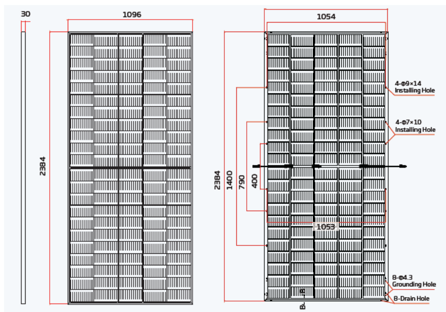
Ilustración 3. Dimensión módulo
