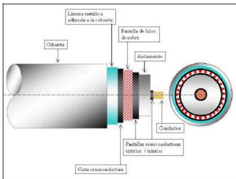
Ilustración 8. Composición conductor
