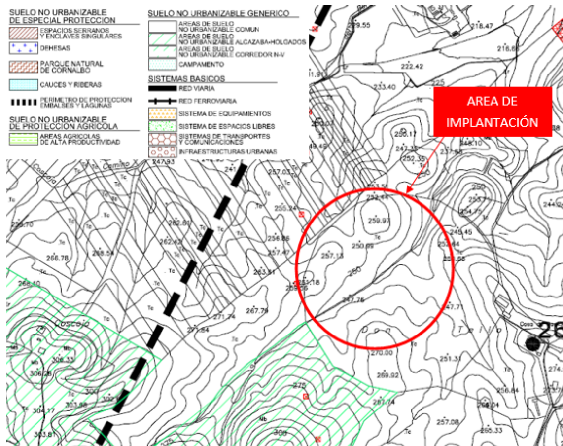
Área de implantación BESS Parque 1
