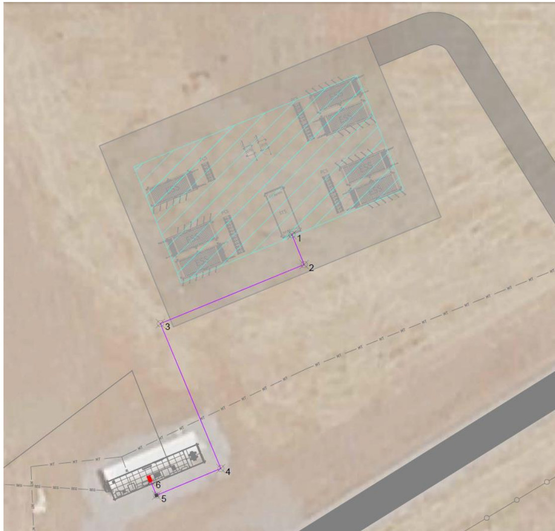
Zanja MT hasta Centro de Seccionamiento
