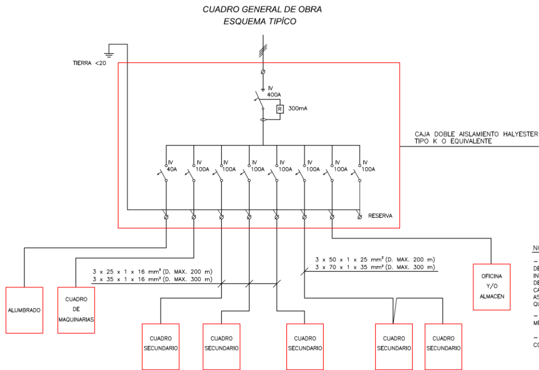
ESQUEMA DE INSTALACIÓN ELÉCTRICA PARA UNA OBRA MEDIANA
