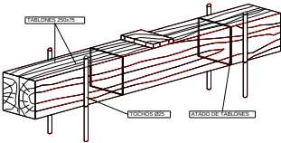
DETALLE DE CALZO
