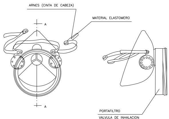
SECCION A-A
