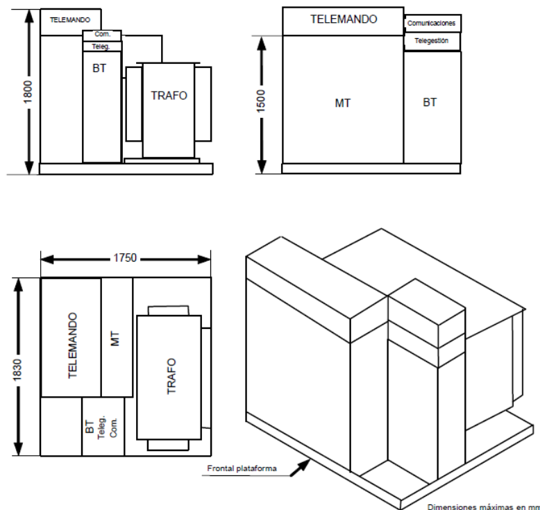
Conjunto compacto para centros de transformación (CTC)
