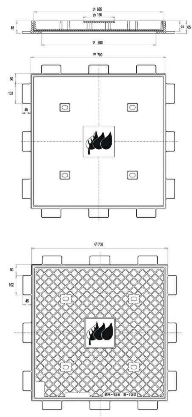
TOI FRANCIA EN TODAS LAS COTAS CON ± 3 mm Detalle Marco M2 y tapa T2 (Dimensiones en mm.)
