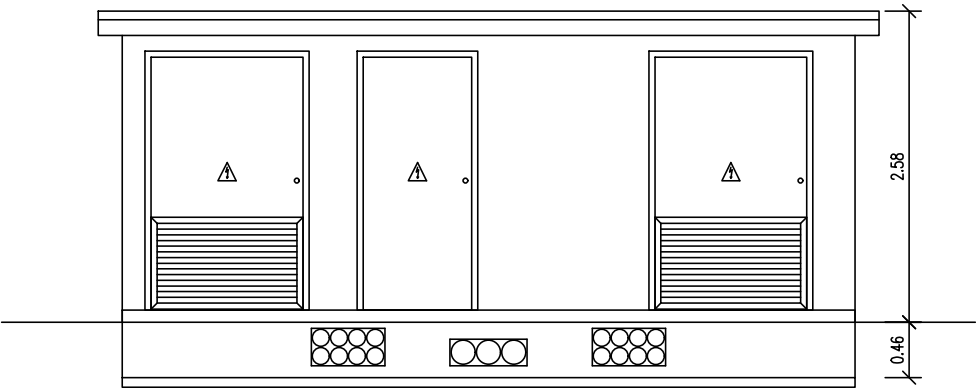
ALZADO FRONTAL
