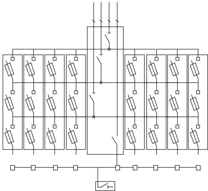
ESQUEMA ELECTRICO
