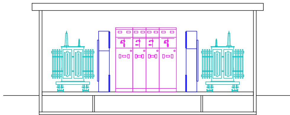
SECCIÓN TRANSVERSAL
