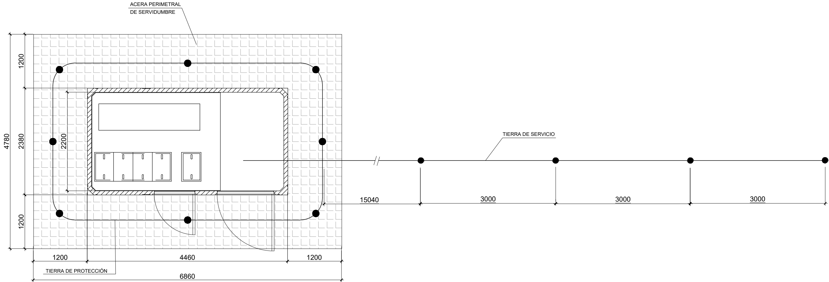
PLANTA
