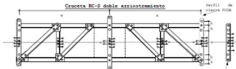
Cruceta RC-S simple arriostramiento
