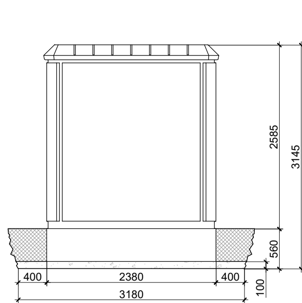
VISTA LATERAL
