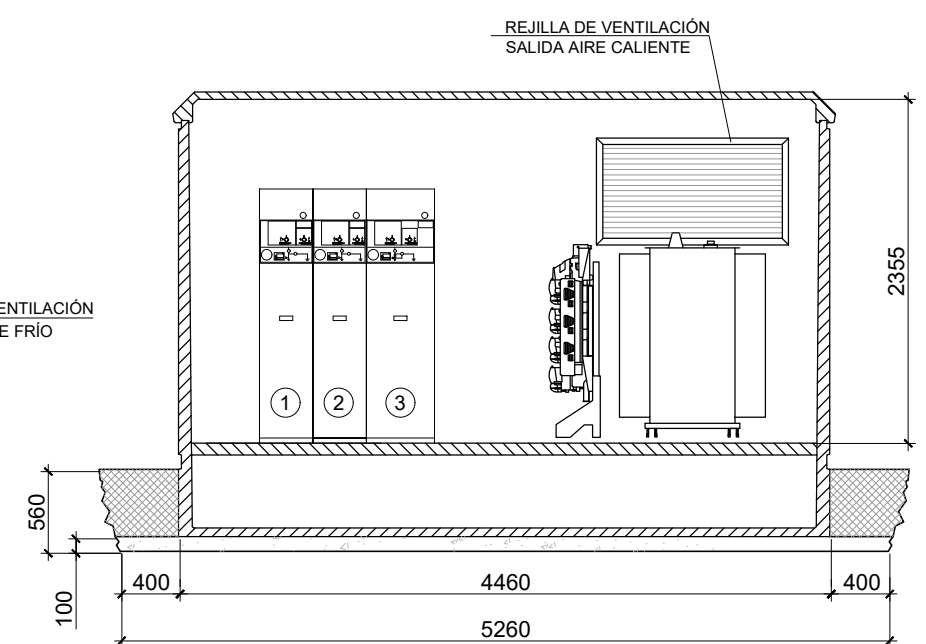
SECCIÓN A-A'
