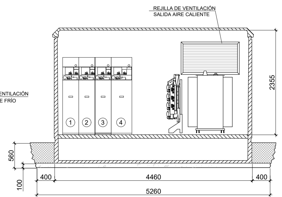
SECCIÓN A-A'
