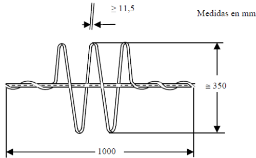
Balizamiento de líneas aéreas mediante espirales
