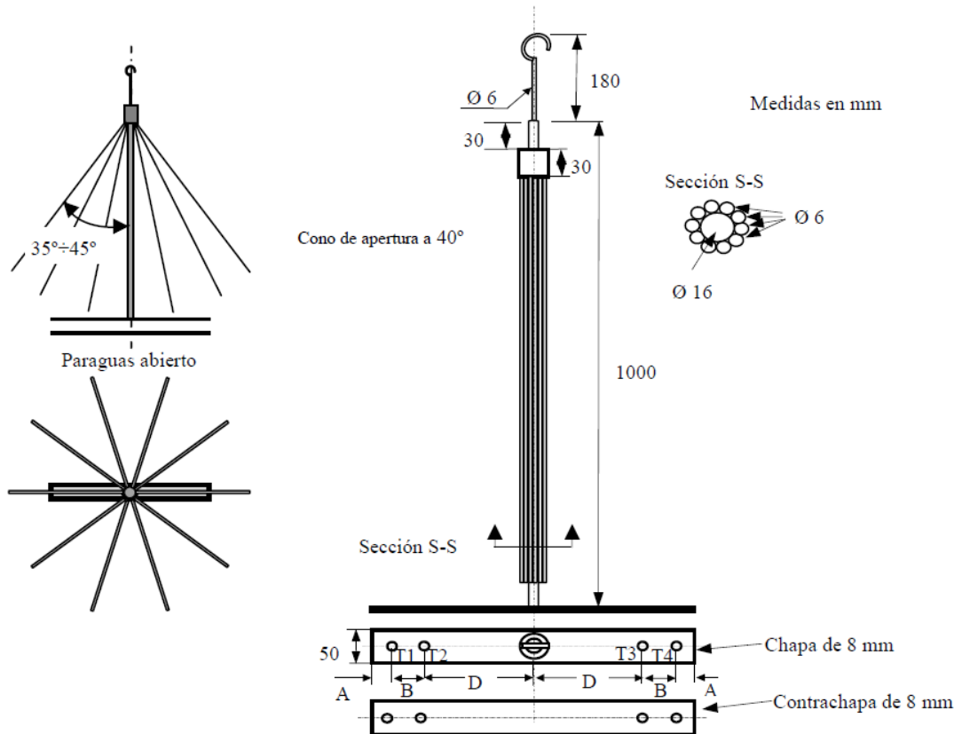
Detalle paraguas metálico 'PAME'
