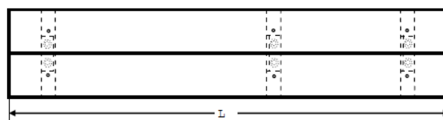
Detalle tejadillos antinidificación para crucetas TACR
