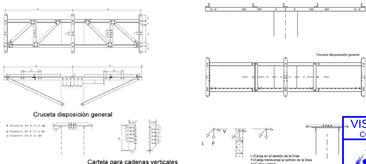
Detalle cruceta recta atirantada 'RC3' y cruceta recta sin atirantar 'RC2'
