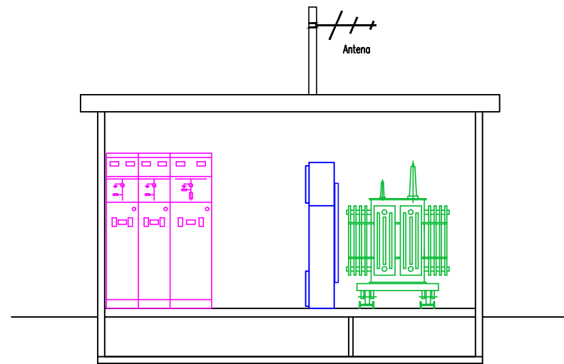
SECCIÓN TRANSVERSAL
