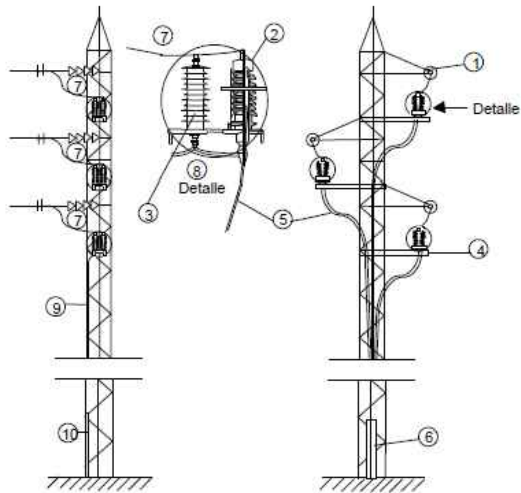
ENTRONQUE AÉREO SUBTERRÁNEO. SIMPLE CIRCUITO
