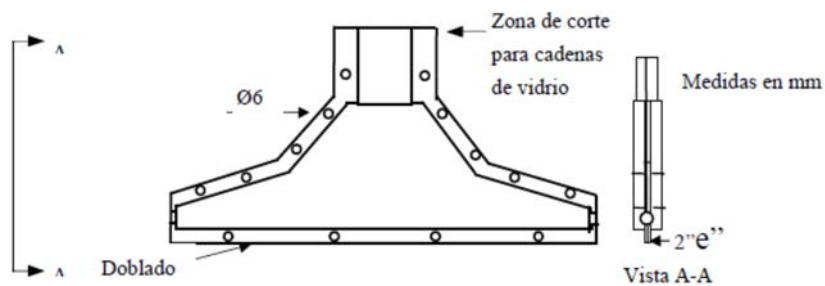
Forros para grapas de suspensión
