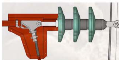
Forros para grapas de amarre a compresión
