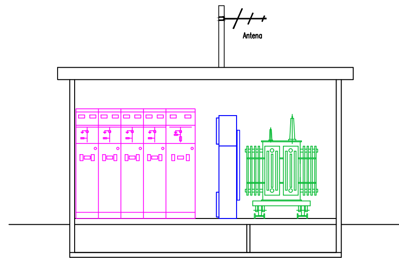
SECCIÓN TRANSVERSAL
