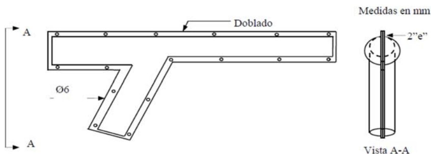
Forros para grapas de amarre a compresión
