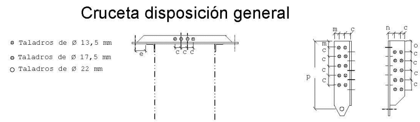
Cartela para cadenas verticales
