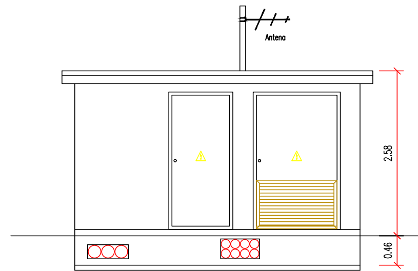
ALZADO FRONTAL
