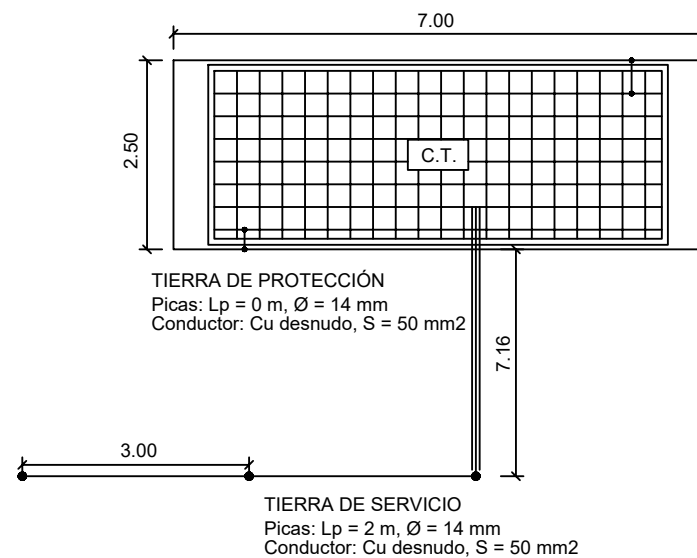
PUESTAS A TIERRA
