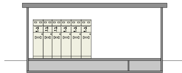
SECCIÓN TRANSVERSAL
