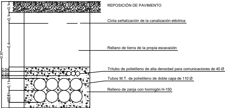
ZANJA DE M.T. ACERADO
