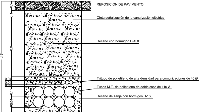
ZANJA DE M.T. CRUCE DE CALZADA
