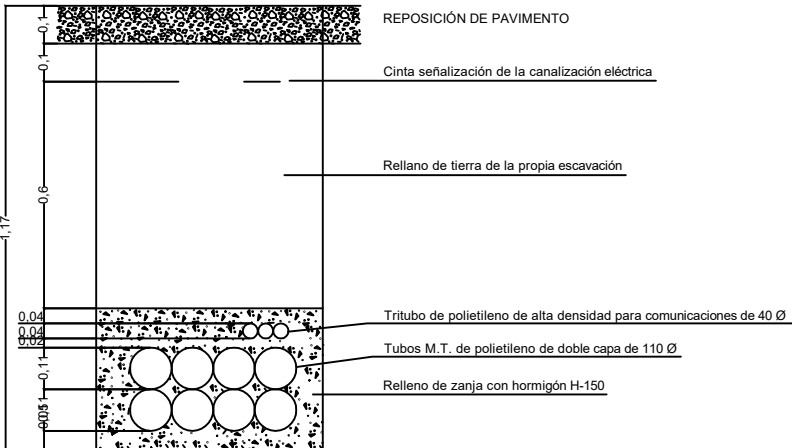
ZANJA DE M.T. CALZADA
