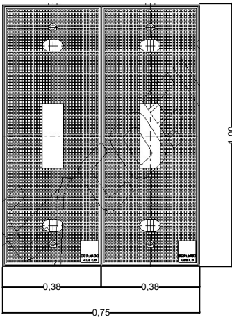
MARCO Y DOS TAPAS REFORZADAS
