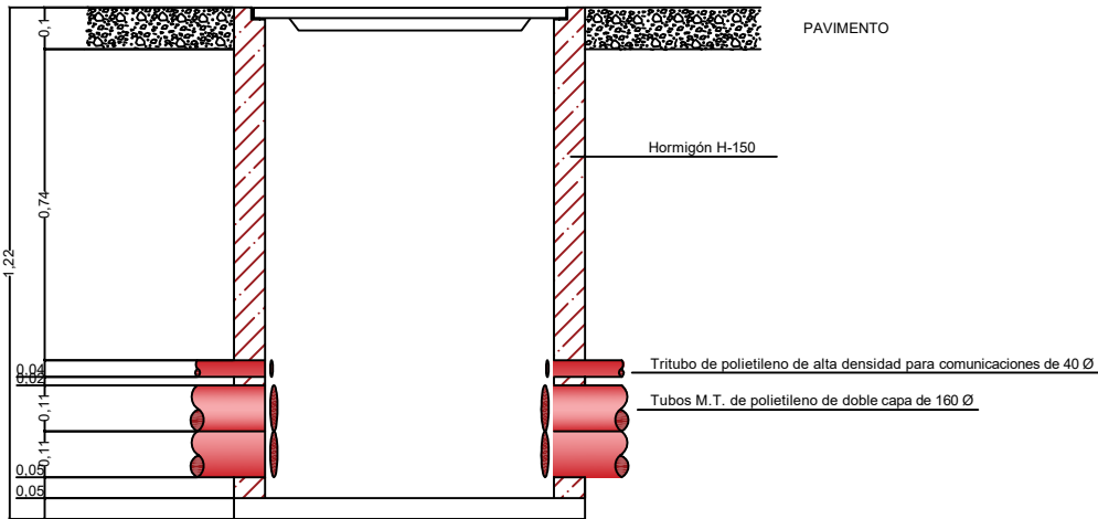
ARQUETA DE DOS TAPAS
