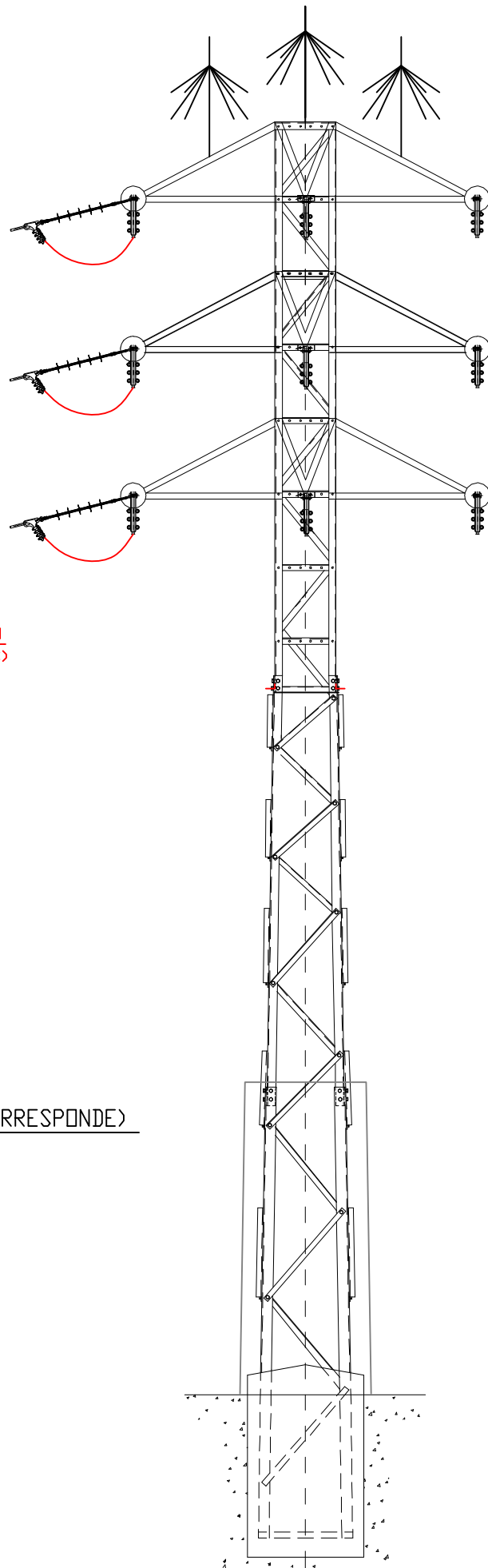
VISTA LATERAL
