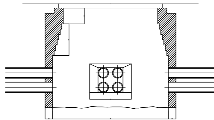
SECCION A-A
