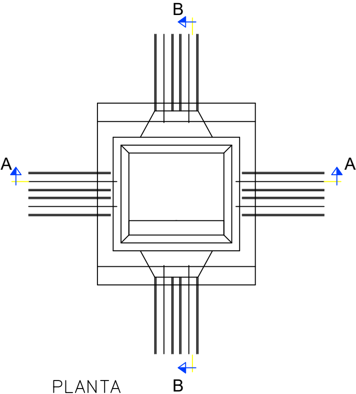
ARQUETA TIPO A-1
