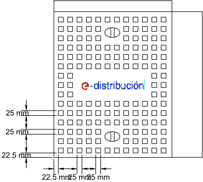
DETALLE 2
