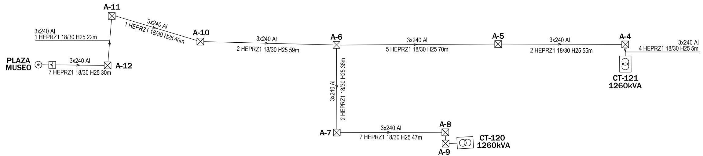
PLANTA
