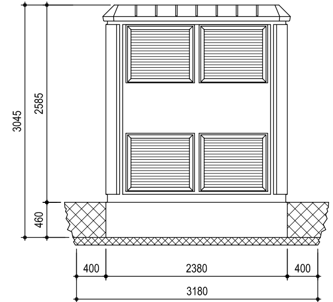
ALZADO LATERAL
