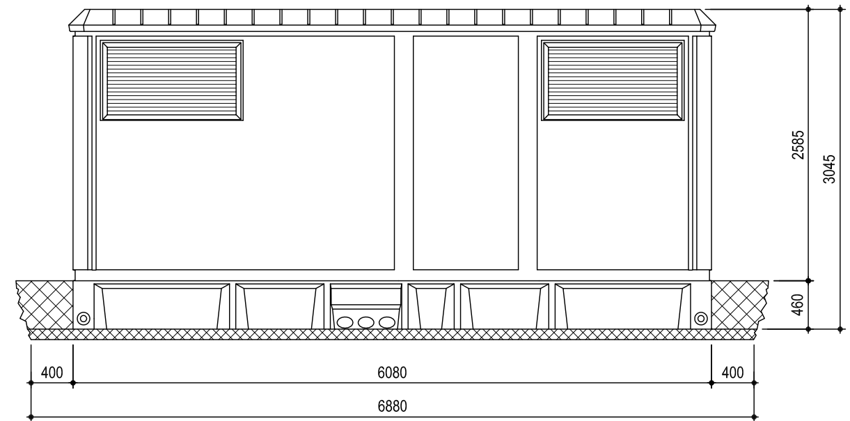
ALZADO POSTERIOR
